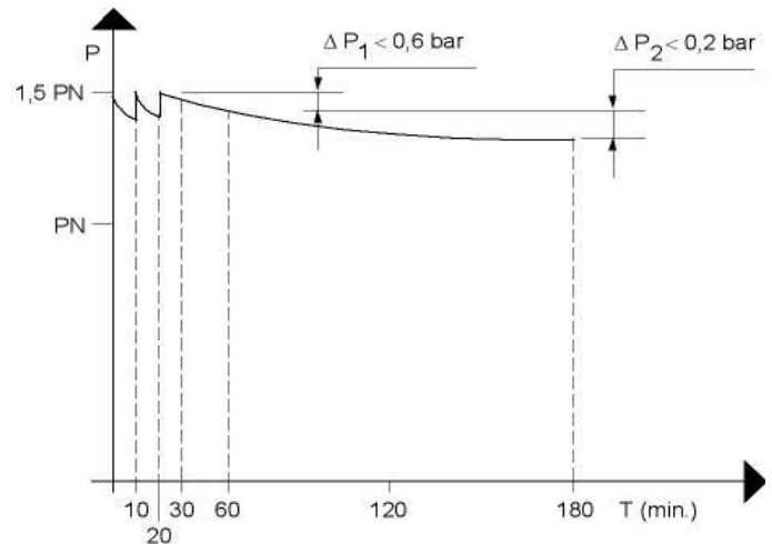
Figure 1 — Contrôle d'étanchéité
