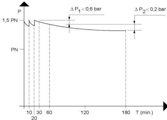
Fig. 1 – Dichtheidscontrole
