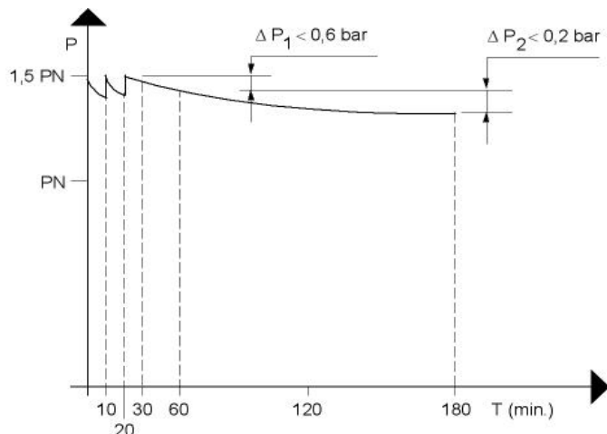
Fig. 1: – Dichtheidscontrole
