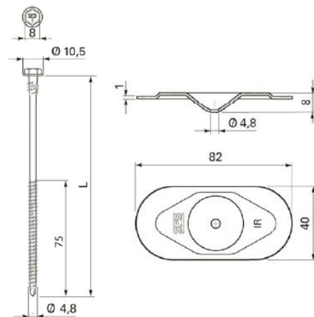
Fig. 3: Vis SFS IR2 4,8 + plaque SFS IR 82x40
