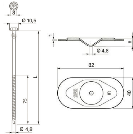
Fig. 3 – Schroef SFS IR2 4,8 + bevestigingsplaatje SFS IR 82X40
