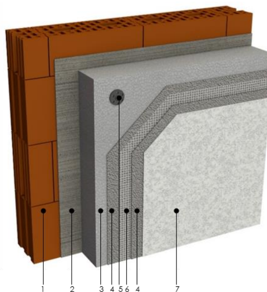
1. Support; 2. Adhésif; 3. Isolation; 4. Enduit de base; 5. (éventuelle) fixation mécanique; 6. Tissu d'armature; 7. Enduit de finition.
