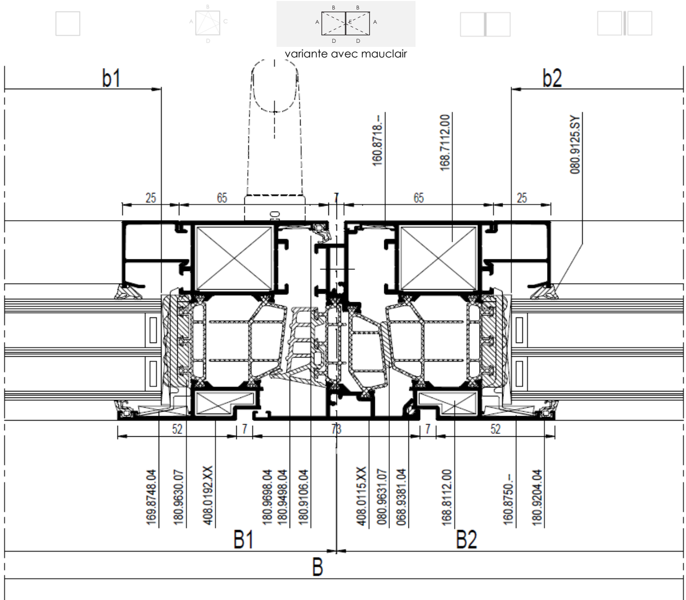
Figure 6 : Coupe-type de fenêtre à double ouvrant
