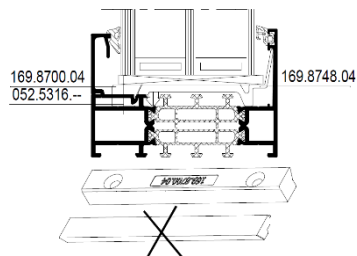
Figure 3 : Variantes d'exécution du support pour cale à vitrage de vantail
