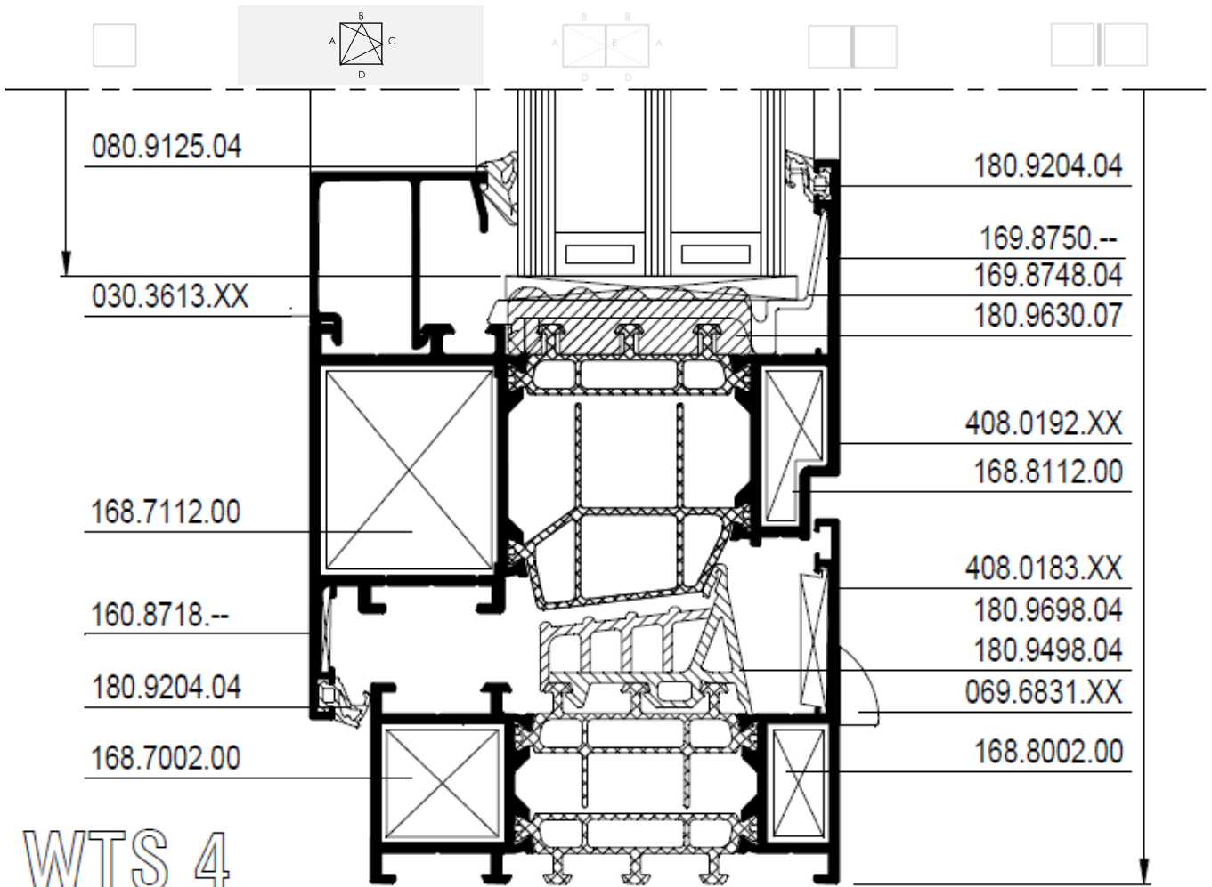
Figure 5 : Coupe-type de fenêtre oscillo-battante
