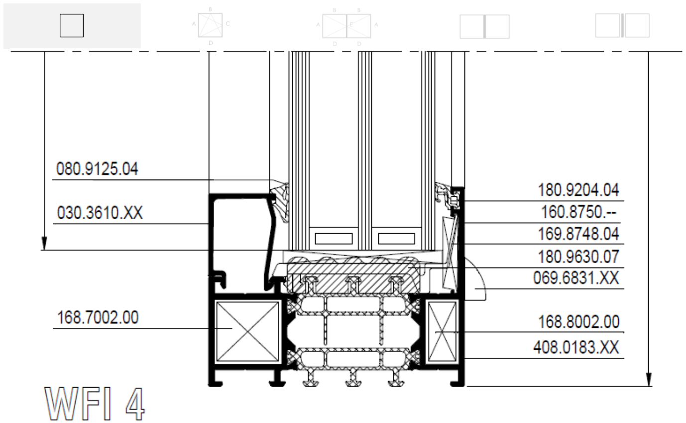
Figure 4 : Coupe-type de fenêtre fixe
