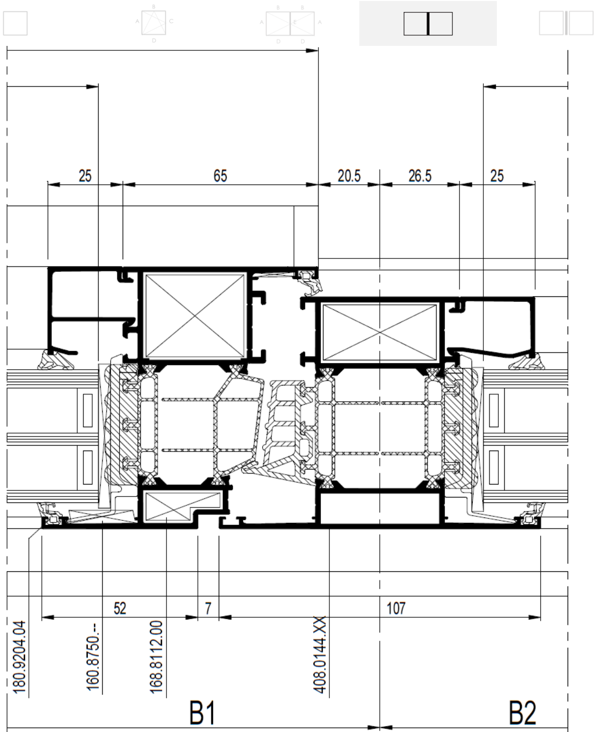
Figure 7 : Coupe-type de fenêtre composée
