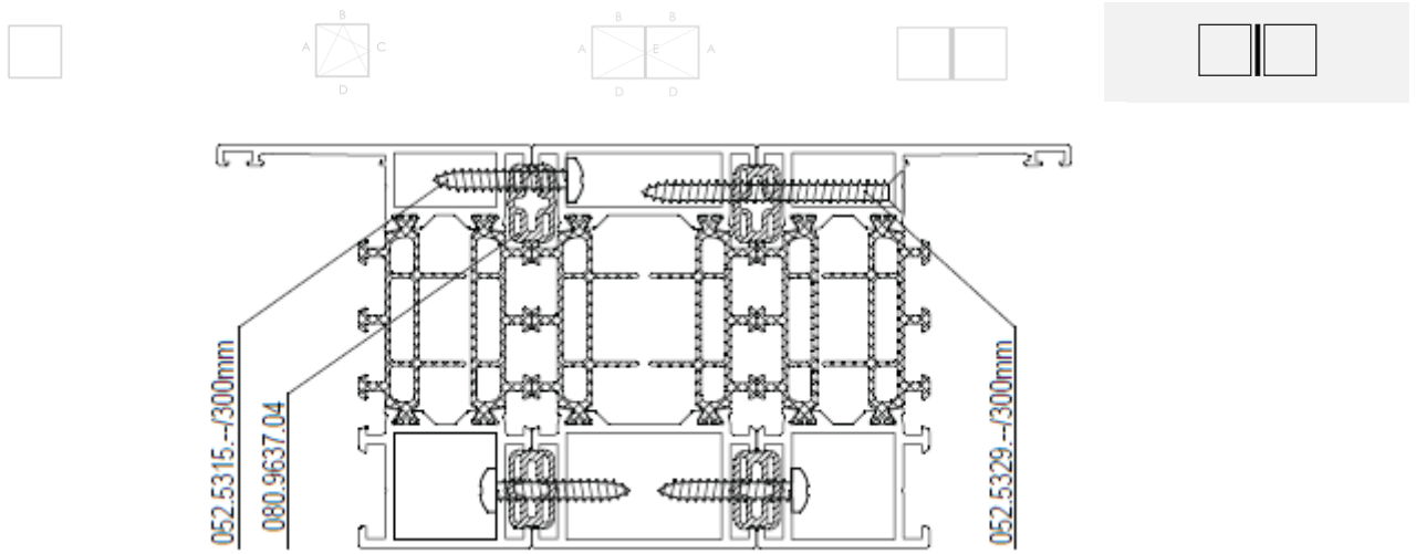
Figure 8 : Coupe-type d'ensemble menuisé
