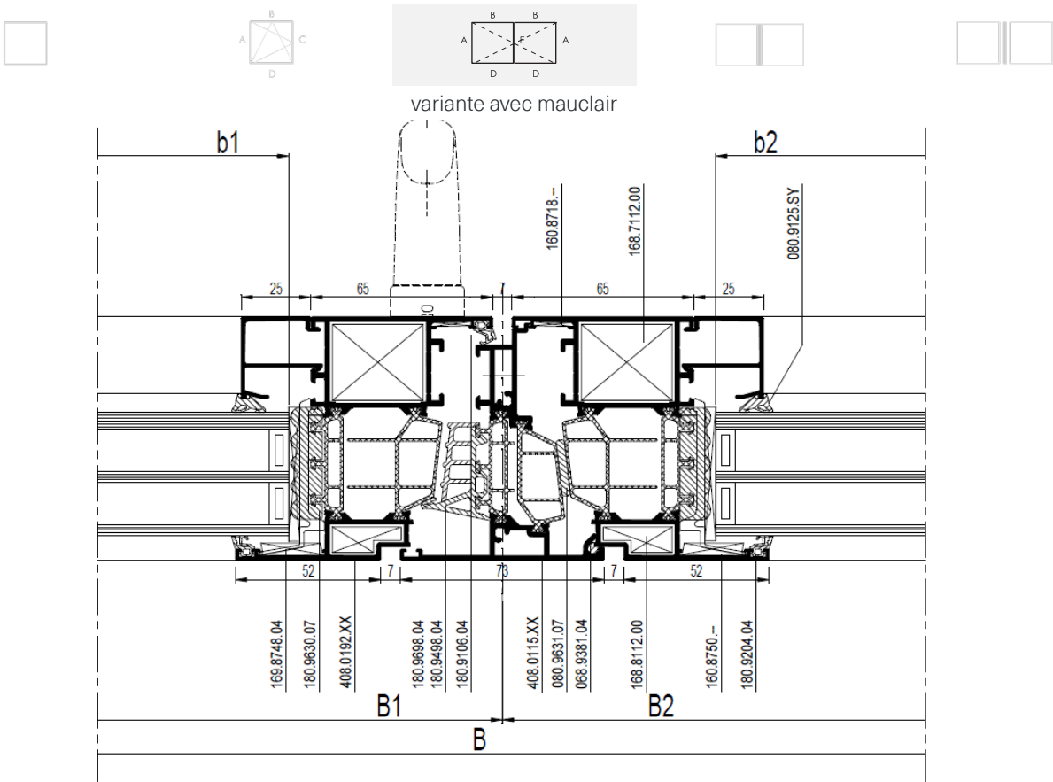
Figure 6 : Coupe-type de fenêtre à double ouvrant
