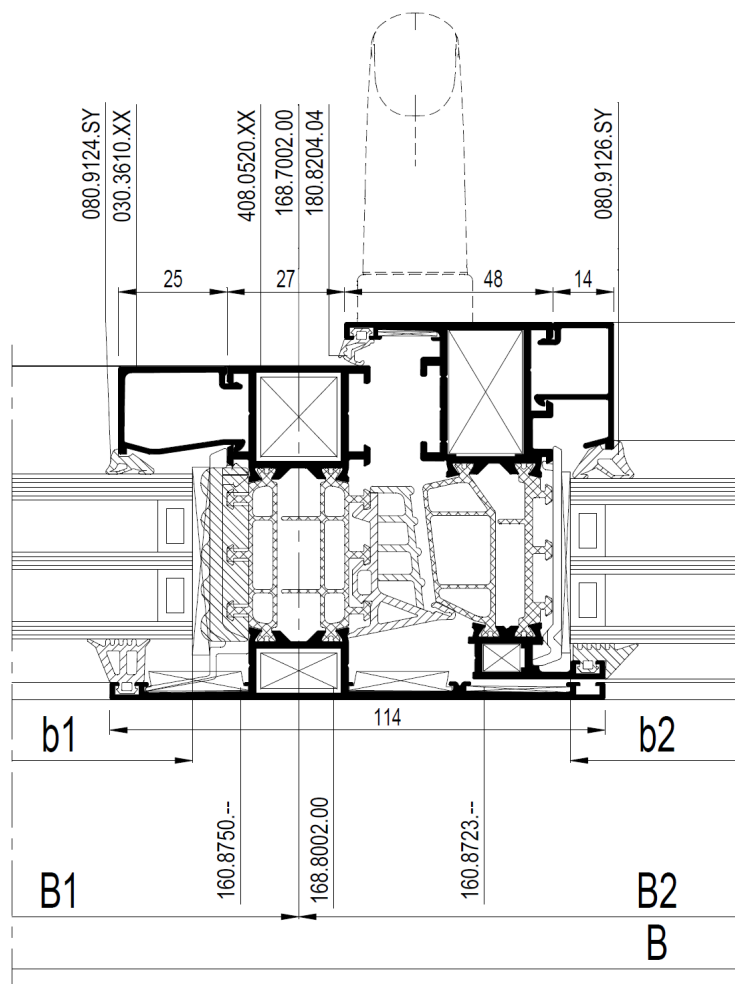
Figure 8 : Coupe-type d'ensemble menuisé
