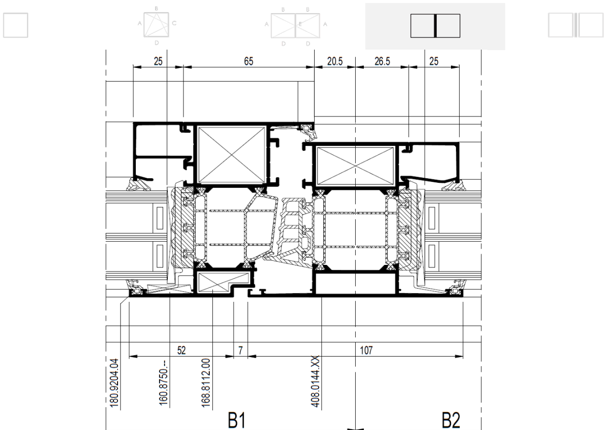
Figure 7 : Coupe-type de fenêtre composée
