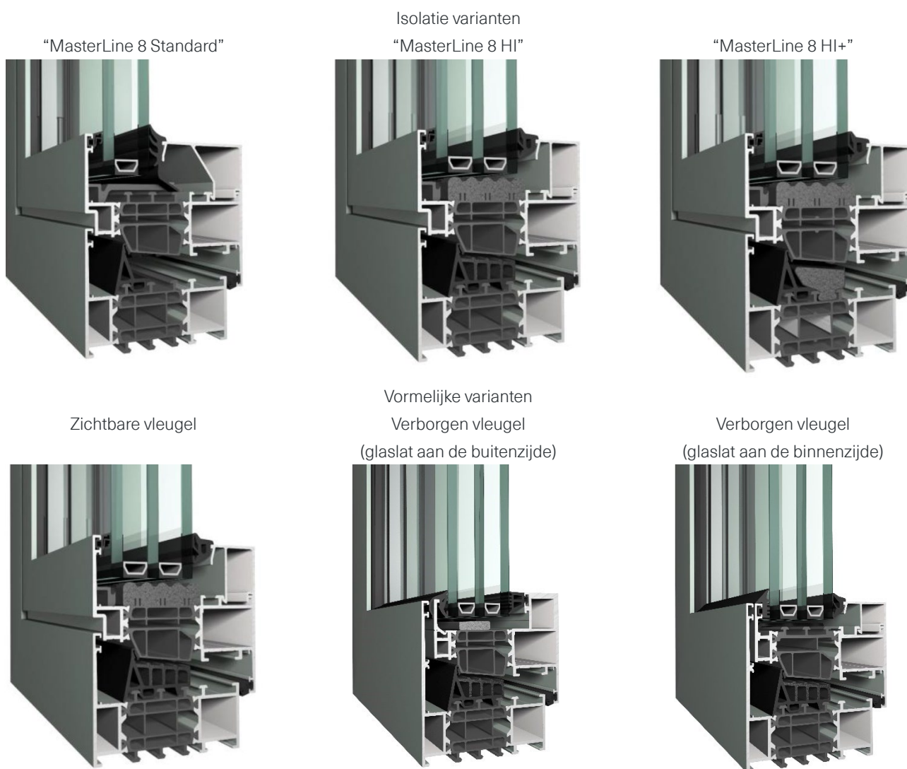
Figuur 1: Uitvoeringsvarianten
