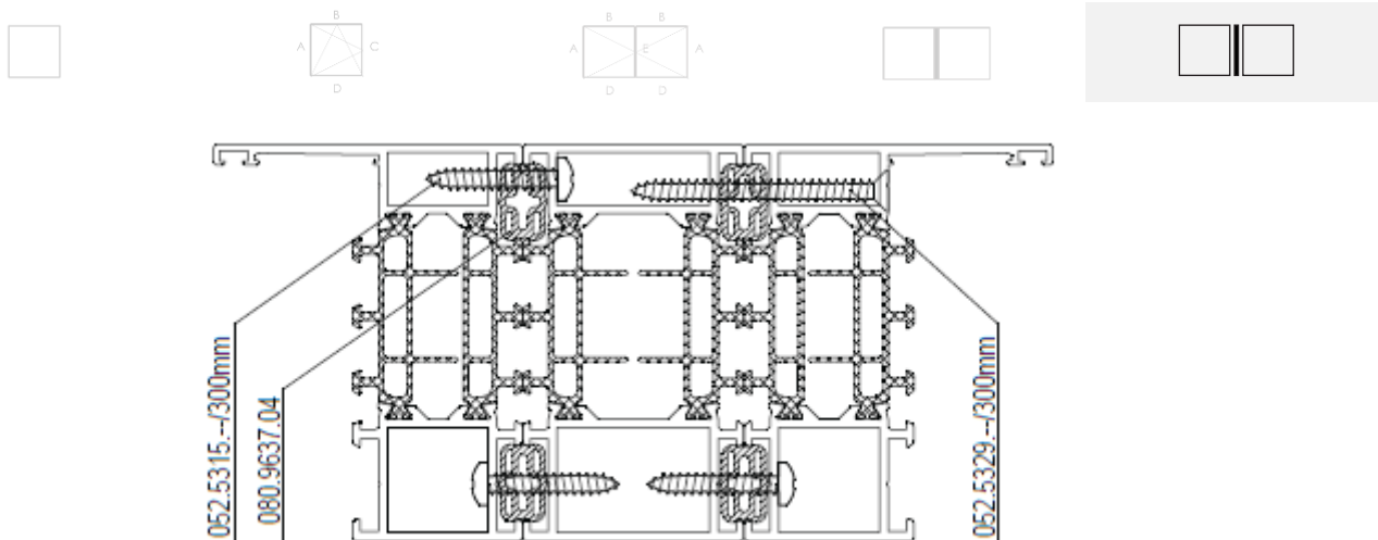
Figuur 8: Typesnede schrijnwerkgeheel
