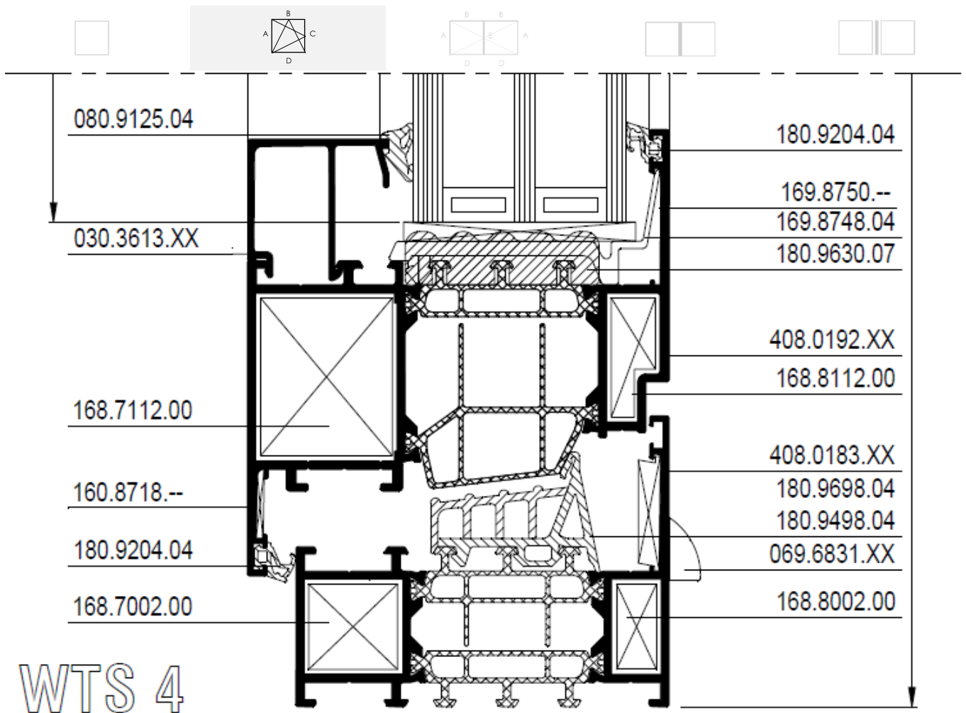
Figuur 5: Typesnede draai-kip venster
