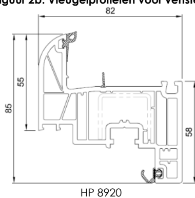
Figuur 2b: Vleugelprofielen voor vensters
