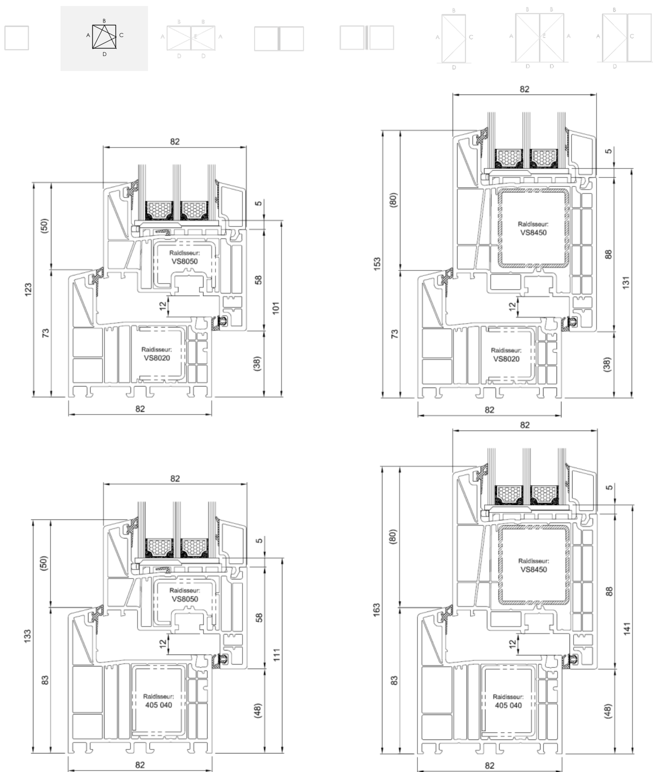
Figuur 7b: Typesnede draai-kip venster
