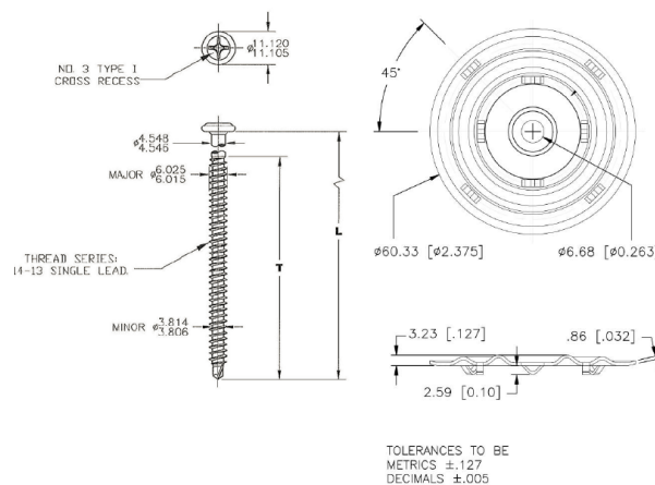
Fig. 1 – Schroef "ALL PURPOSE" FASTENER + bevestigingsplaatje HD SEAM PLATE
