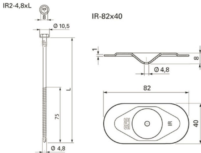
Fig. 2 – Schroef SFS INTEC "IR2-4,8xL" fastener + bevestigingsplaatje "IR-82x40"
