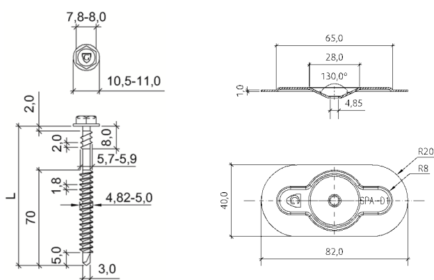
Fig. 4 – Schroef GUARDIAN DBT(A) + bevestigingsplaatje GUARDIAN SPA 8240
