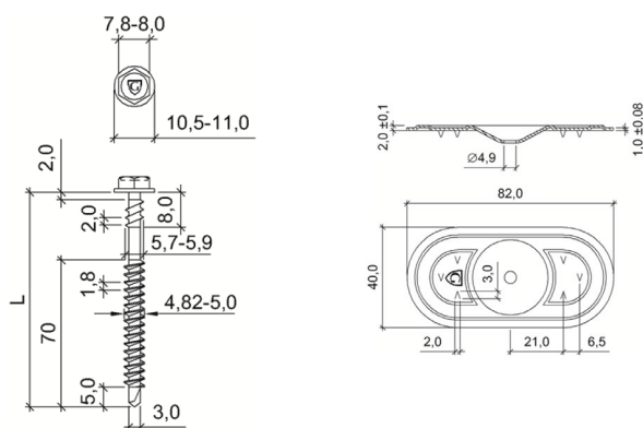
Fig. 5 – Schroef GUARDIAN DBT(A) + bevestigingsplaatje GUARDIAN SPBA 8240
