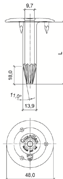
Fig. 8 – Bevestigingsplaatje GUARDIAN RB 48
