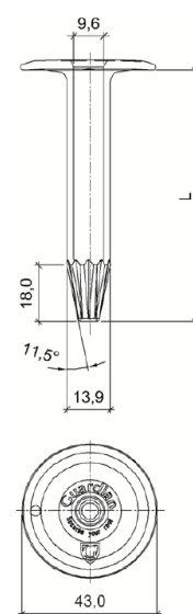
Fig. 7 – Bevestigingsplaatje GUARDIAN SP 50
