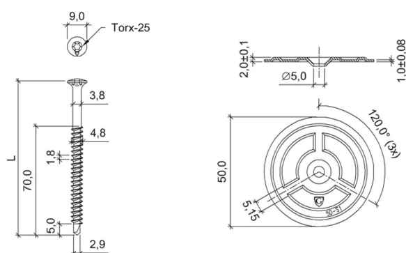
Fig. 6 – Schroef GUARDIAN BS 48
