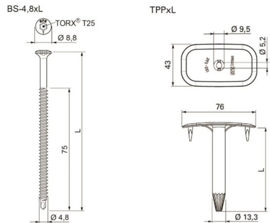
Fig. 3 – Schroef SFS INTEC ISOTAK BS-4,8xL + bevestigingsplaatje ISOTAK TWIN PEAK PLUS TPP 8040
