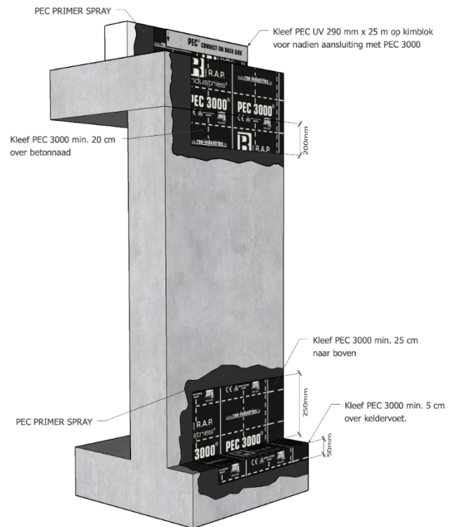
Fig. 4 – Toepassing PEC 3000® op gegoten of prefab betonnen kelder
