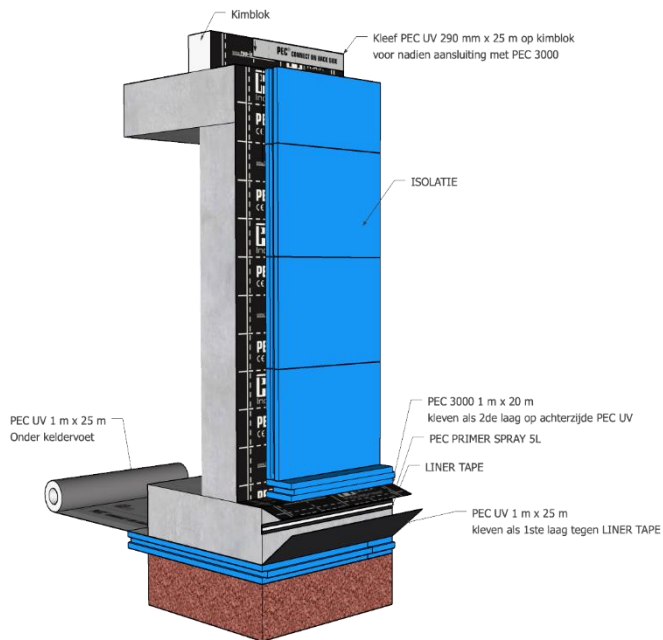
Fig. 5 – Toepassing PEC 3000® op gegoten of prefab betonnen kelder met harde isolatieplaat
