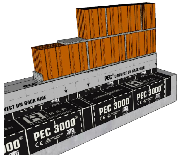
Fig. 8 – uitvoering van PEC® UV als waterkerend membraan in de kimlaag van het metselwerk
