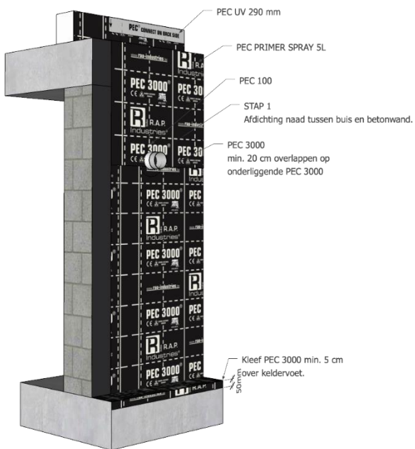
Fig. 9 – Waterdichting ter hoogte van doorvoeren in gemetste kelderwanden
