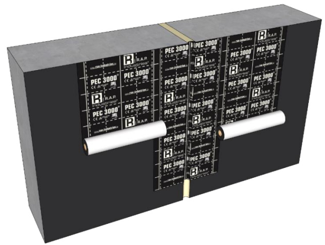
Fig. 7 – Waterdichting ter hoogte van dilatatievoegen
