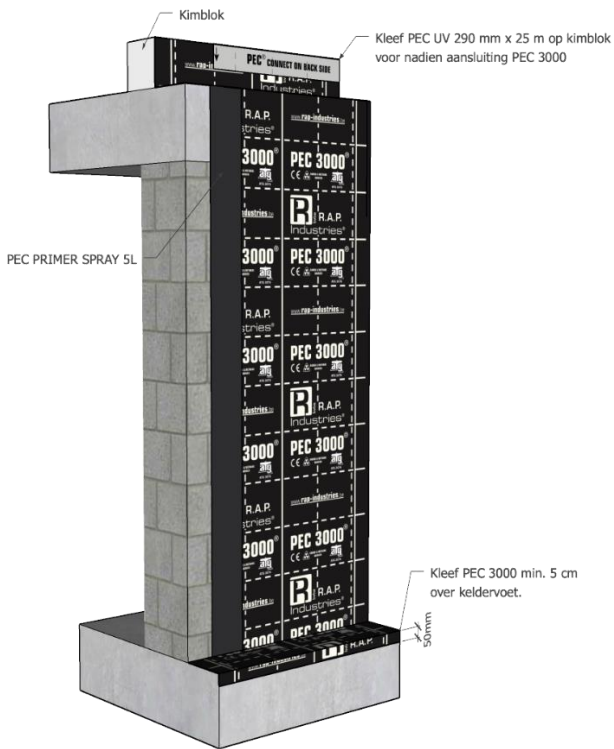
Fig. 6 – Toepassing PEC 3000® op gemetste kelderwand
