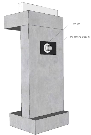
Fig. 10 – Waterdichting ter hoogte van doorvoeren in betonnen elementen
