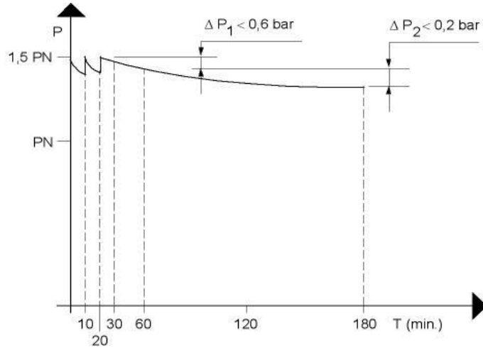
Figure 1 — Contrôle d'étanchéité
