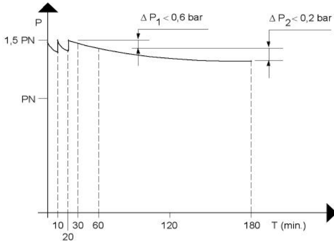
Fig. 1 : Dichtheidscontrole
