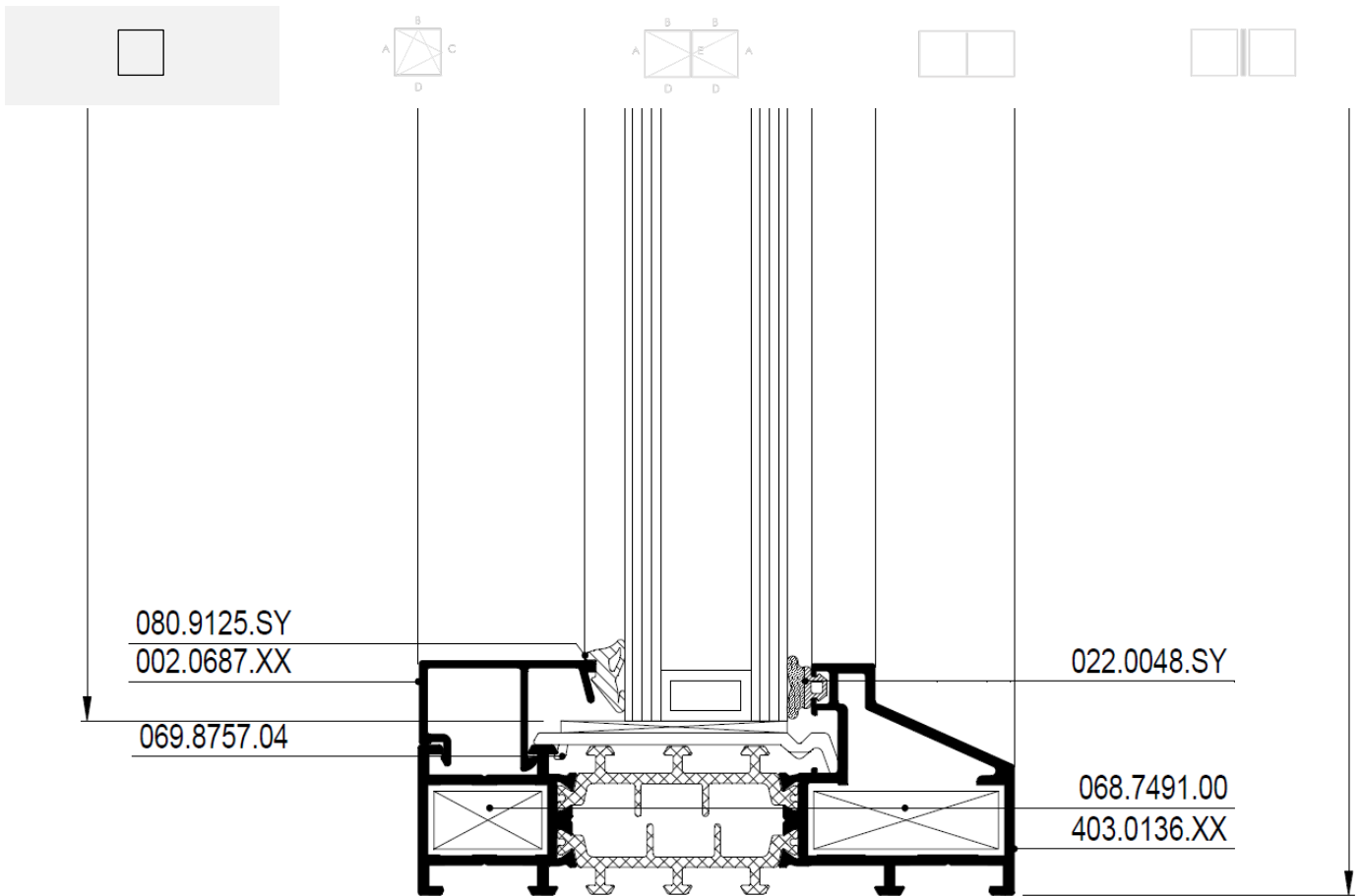
Figure 3 : Coupe-type de fenêtre fixe
