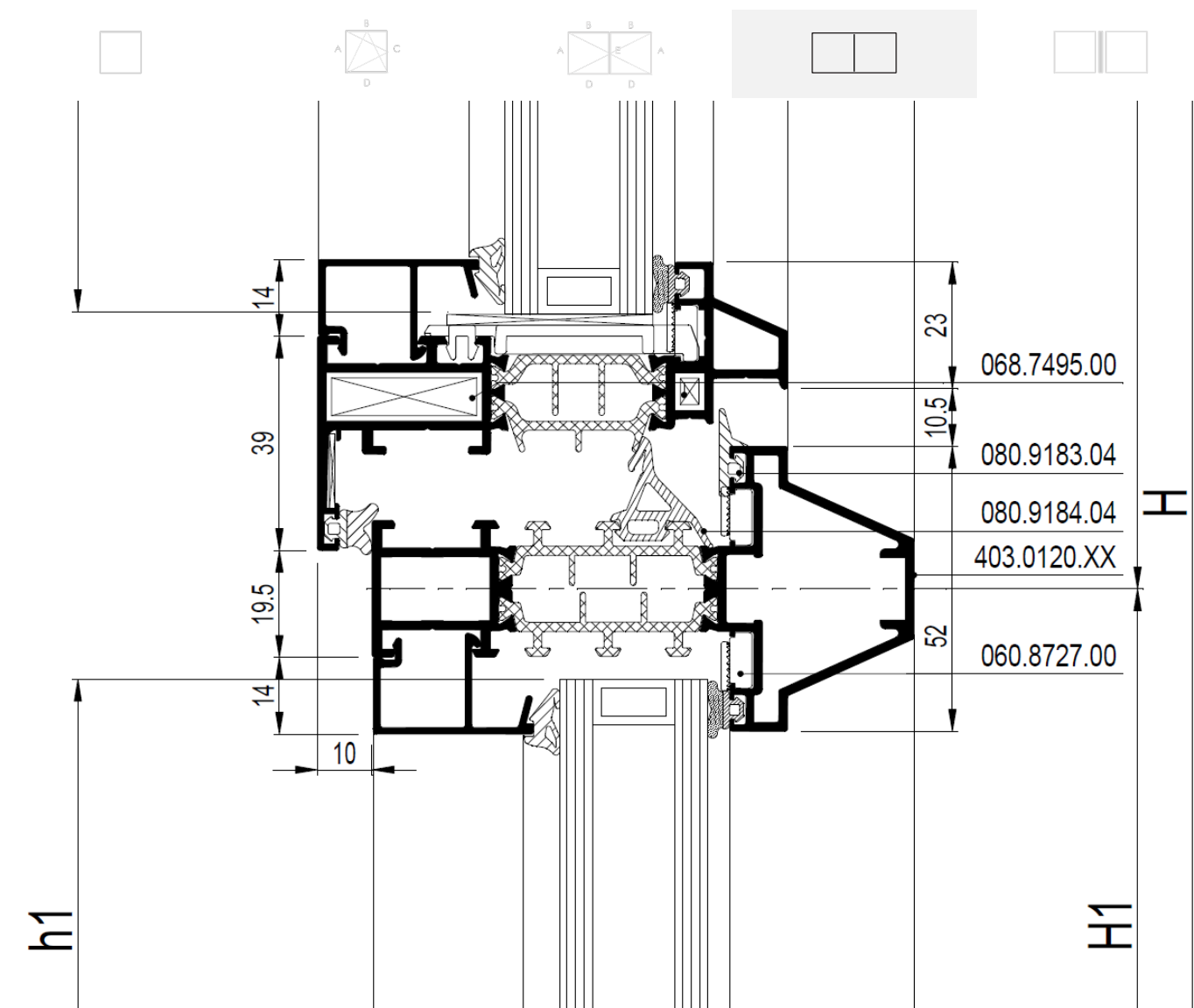
Figure 6 : Coupe-type de fenêtre composée
