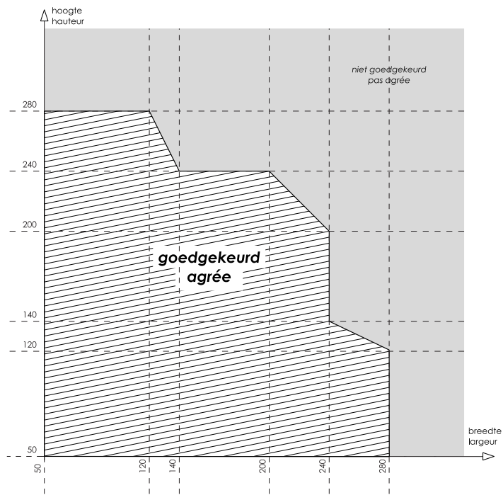
Beslagdiagramma
