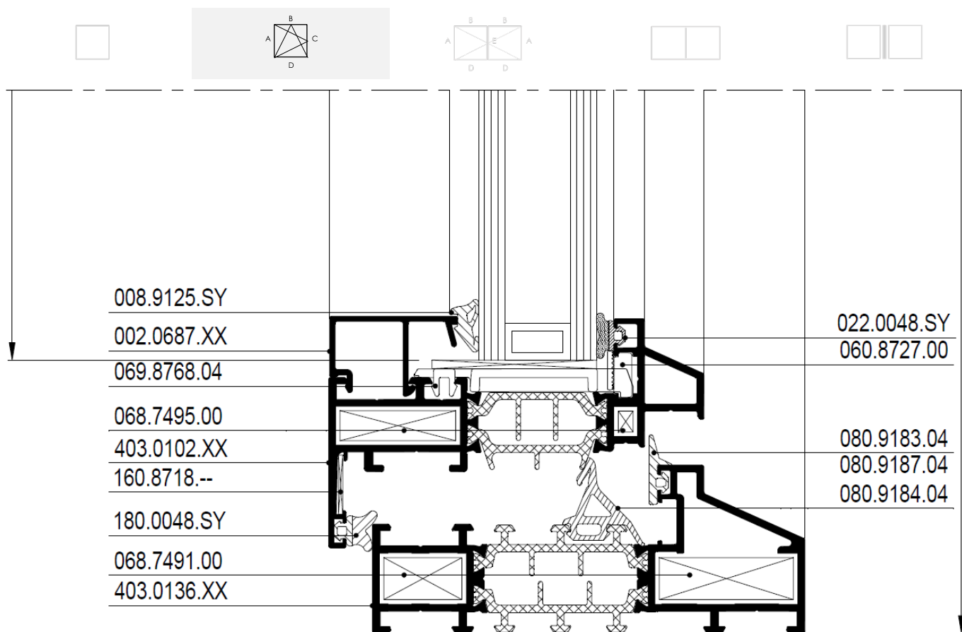
Figuur 4: Typesnede draai-kip venster
