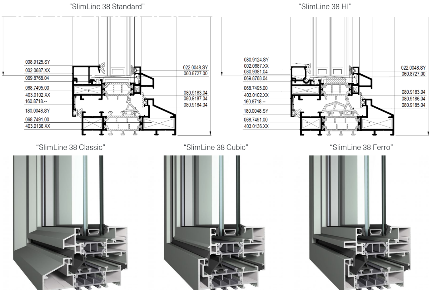
Figuur 2: Uitvoeringsvarianten drager voor glassteunblok
