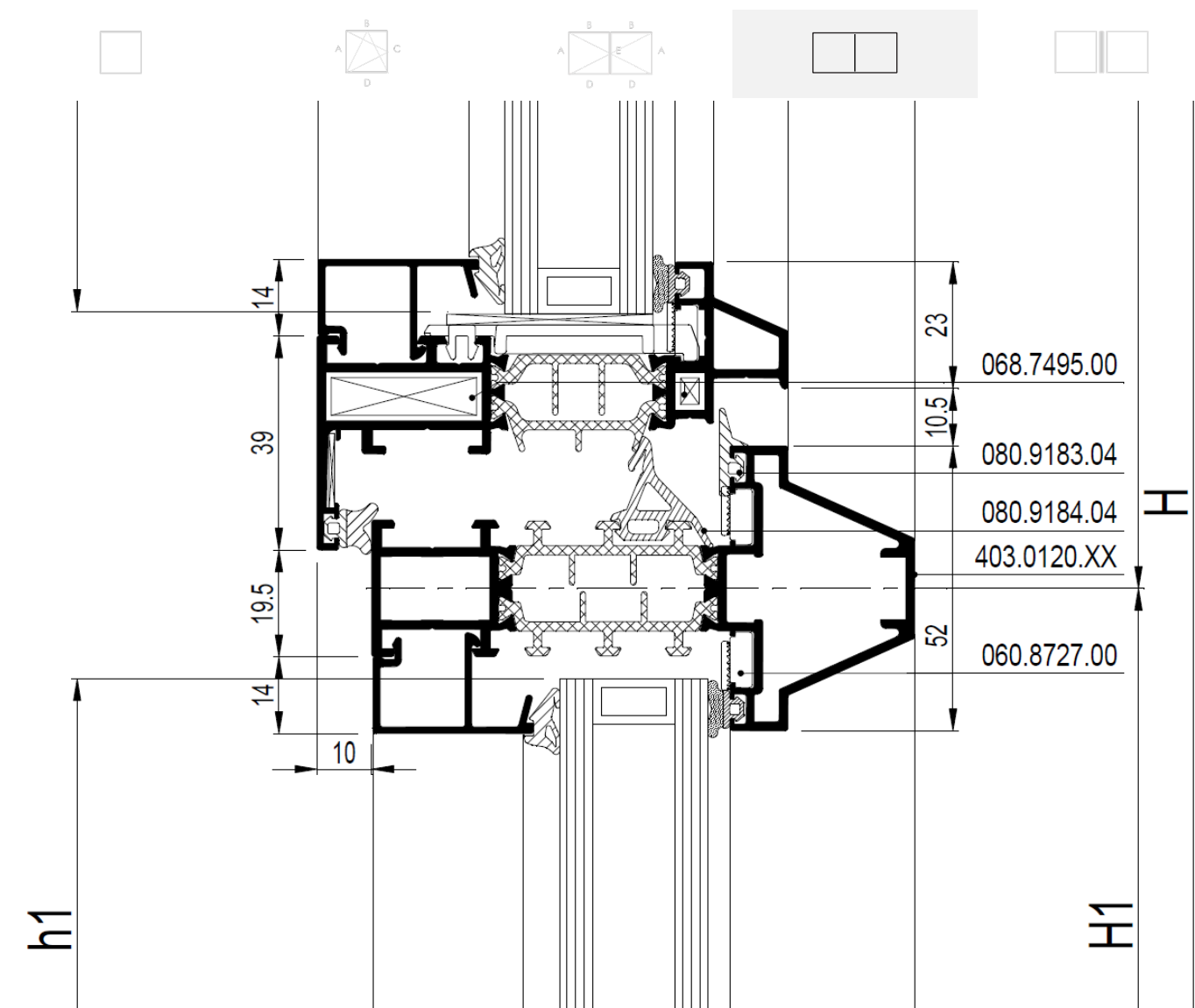
Figuur 6: Typesnede samengesteld venster
