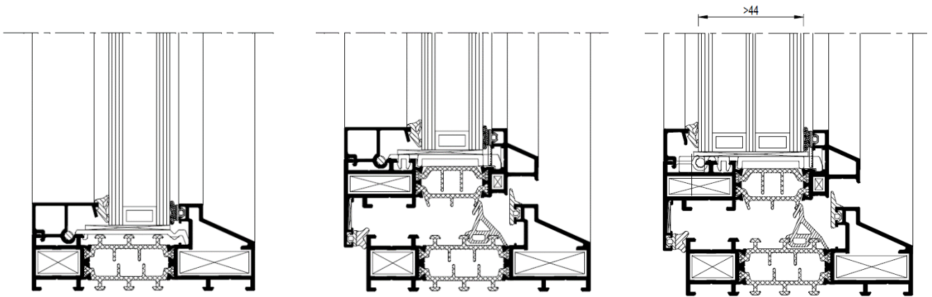
Figuur 3: Typesnede vast venster
