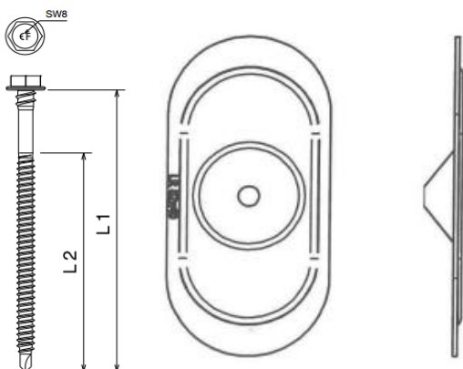
Fig. 1 – Schroef LR ETANCO® EHB DF 2C + bevestigingsplaatje LR ETANCO® 82x40 R DF
