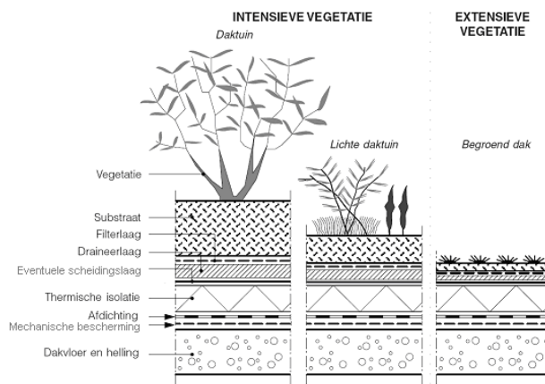
Fig. 2 – Omkeerdak opbouw
