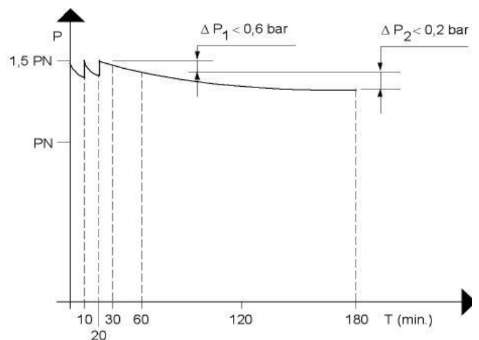
Figuur 2 - Dichtheidscontrole
