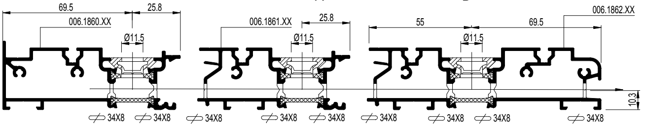
Section D-D
