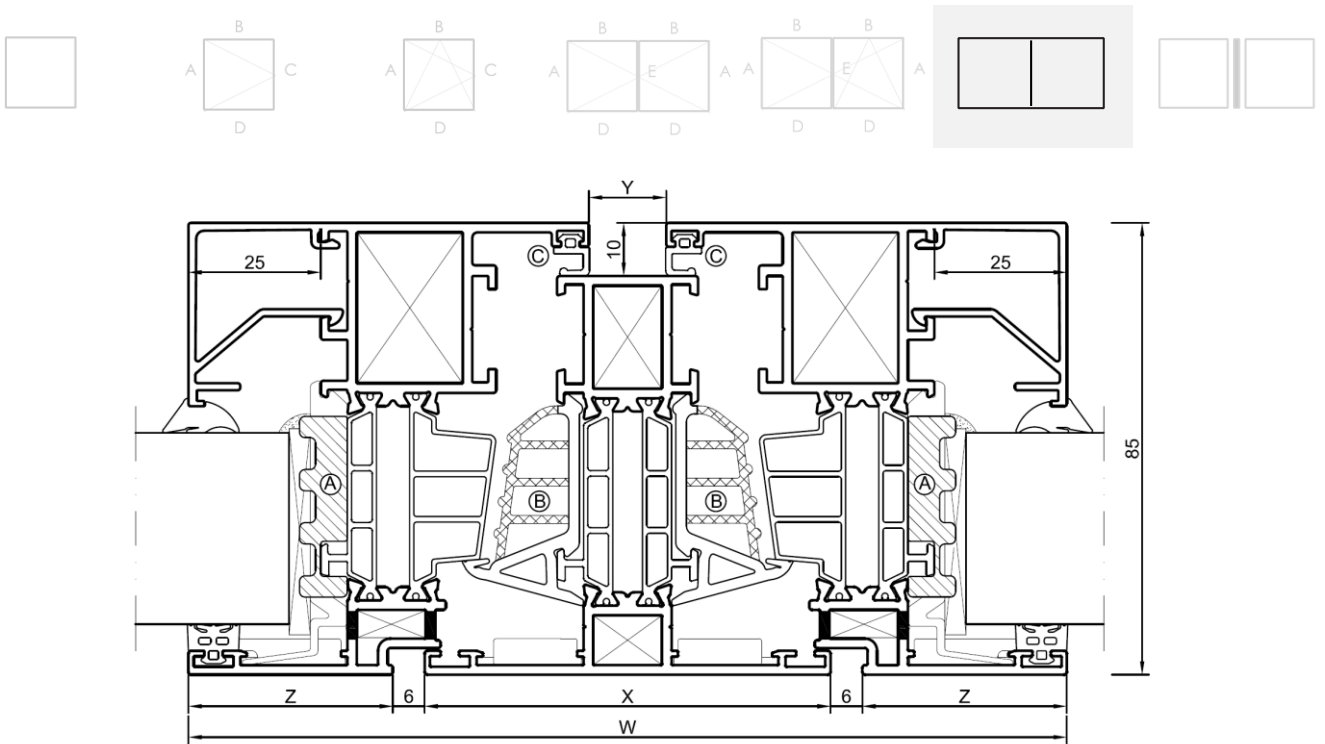
Figure 5 : Coupe-type de fenêtre composée
