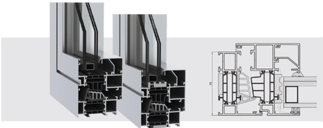
Figuur 1: Uitvoeringsvarianten
