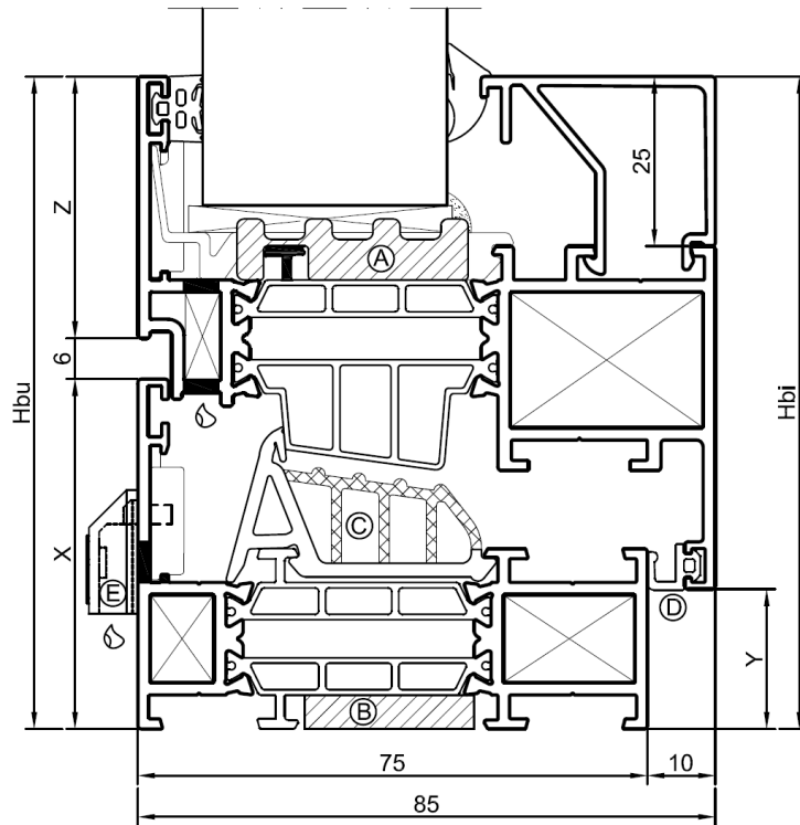
Figuur 3: Uitvoeringsvarianten raai-kip venster
