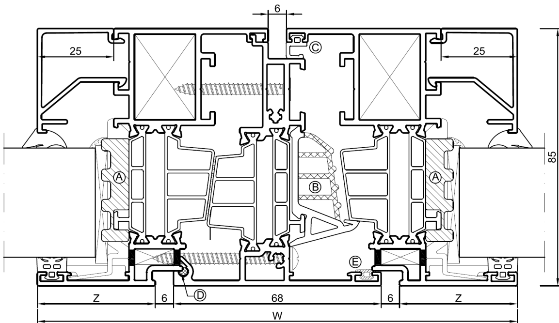
Figuur 4: Uitvoeringsvarianten stolp venster
