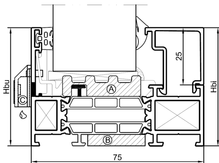
Figuur 2: Uitvoeringsvarianten vast venster
