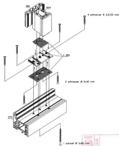
Figure 2d: Assemblage mécanique en T
