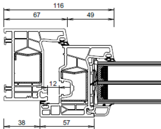
Figure 7b: Coupe-type de fenêtre oscillo-battante
