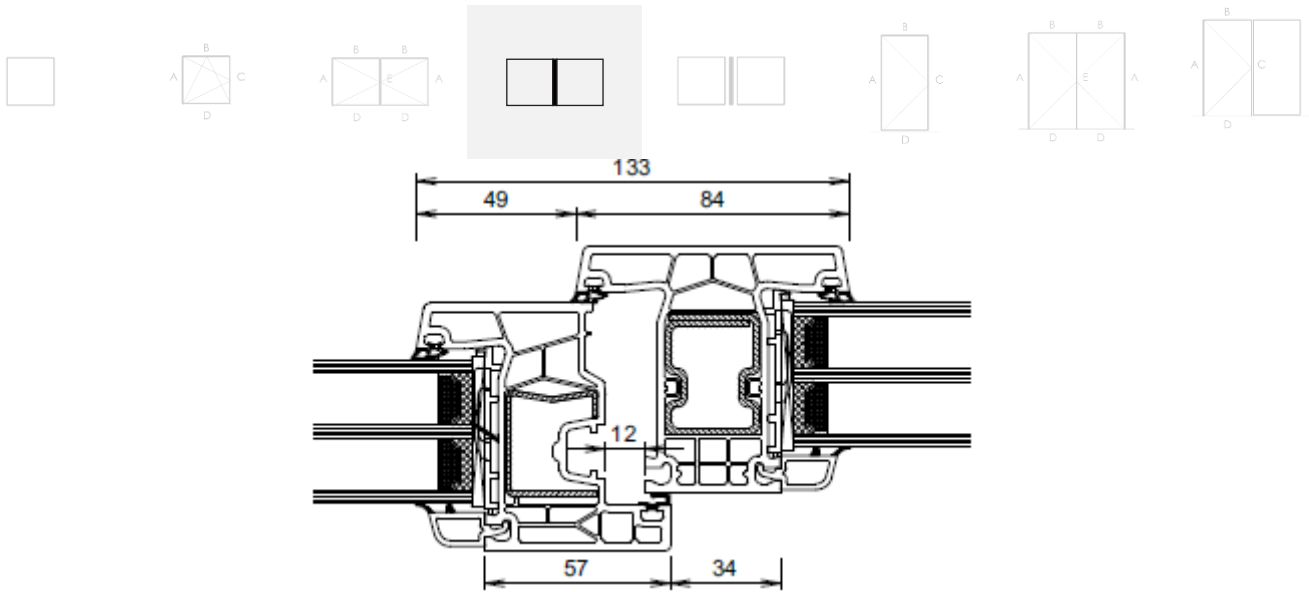
Figure 7d: Coupe-type de fenêtre composée
