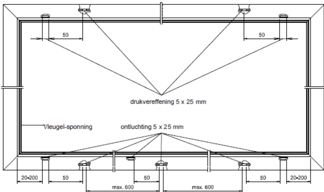
Binnenaanzicht vleugel
