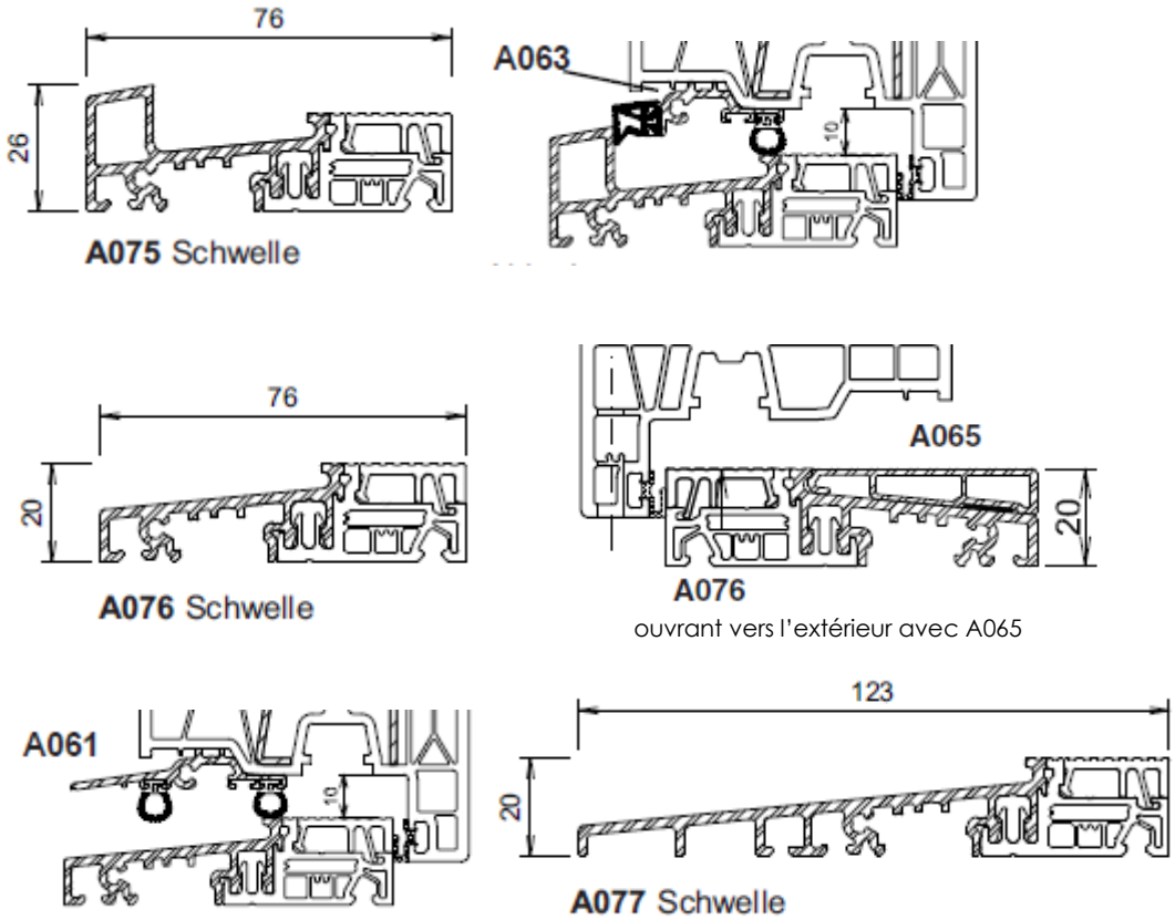
Figure 5.c: seuils de porte en aluminium
