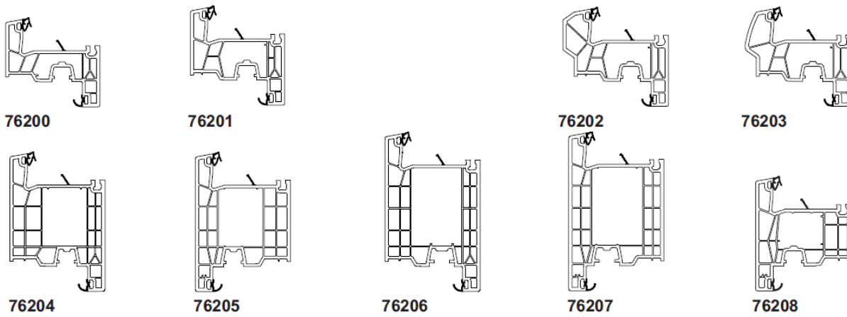
Figure 2c: Montants intermédiaires et traverses
