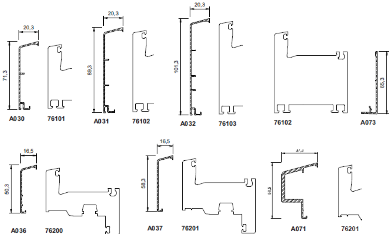
Figure 5b: Couvertres en aluminium sans fonction de résistance
