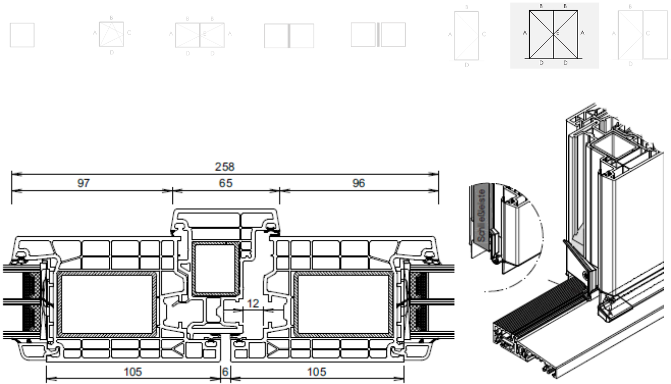
Figure 8b: Coupe-type de porte double ouvrant avec mauclair
