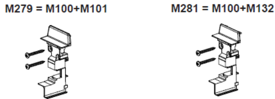
Figure 6.b: Embouts pour maucclair 76401 prévu de couvercle en aluminium
