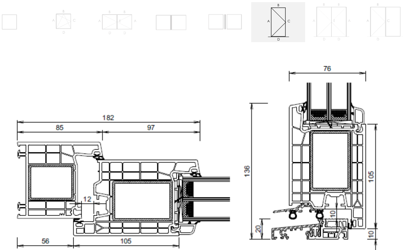
Figure 8a: Coupe-type de porte simple ouvrant (à profilé de frappe)
