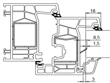
Figure 10 – Séparateur de convection dans la feuillure des profilés
