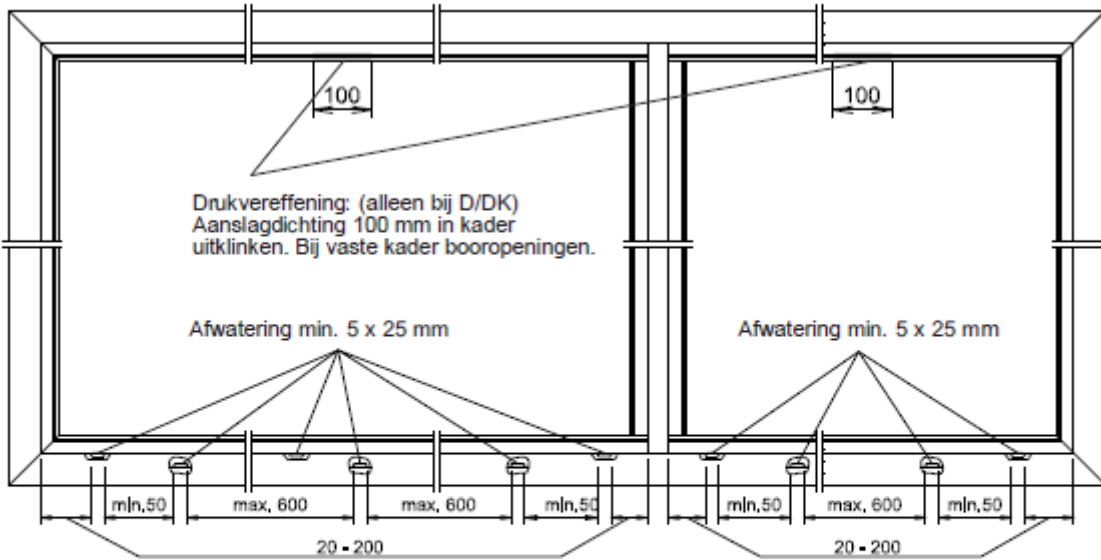
Binnenaanzicht tussenregel
