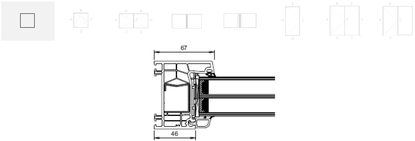
Figure 7a: Coupe-type de fenêtre fixe
