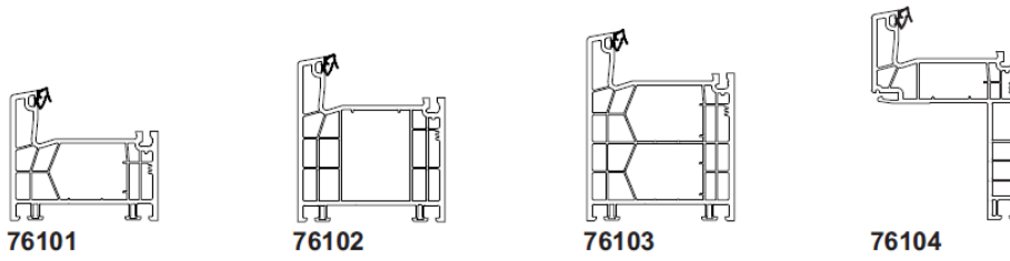
Figure 2b: Profilés d'ouvrant
