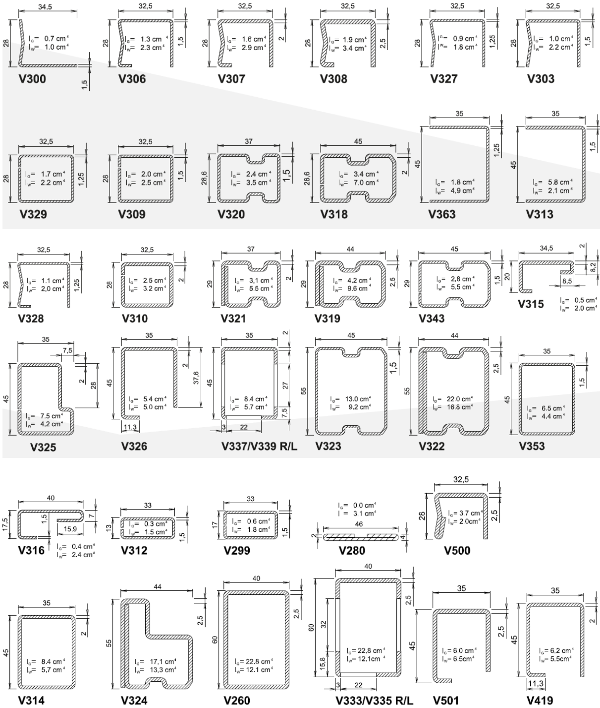
Figure 3: Profilés de renfort
