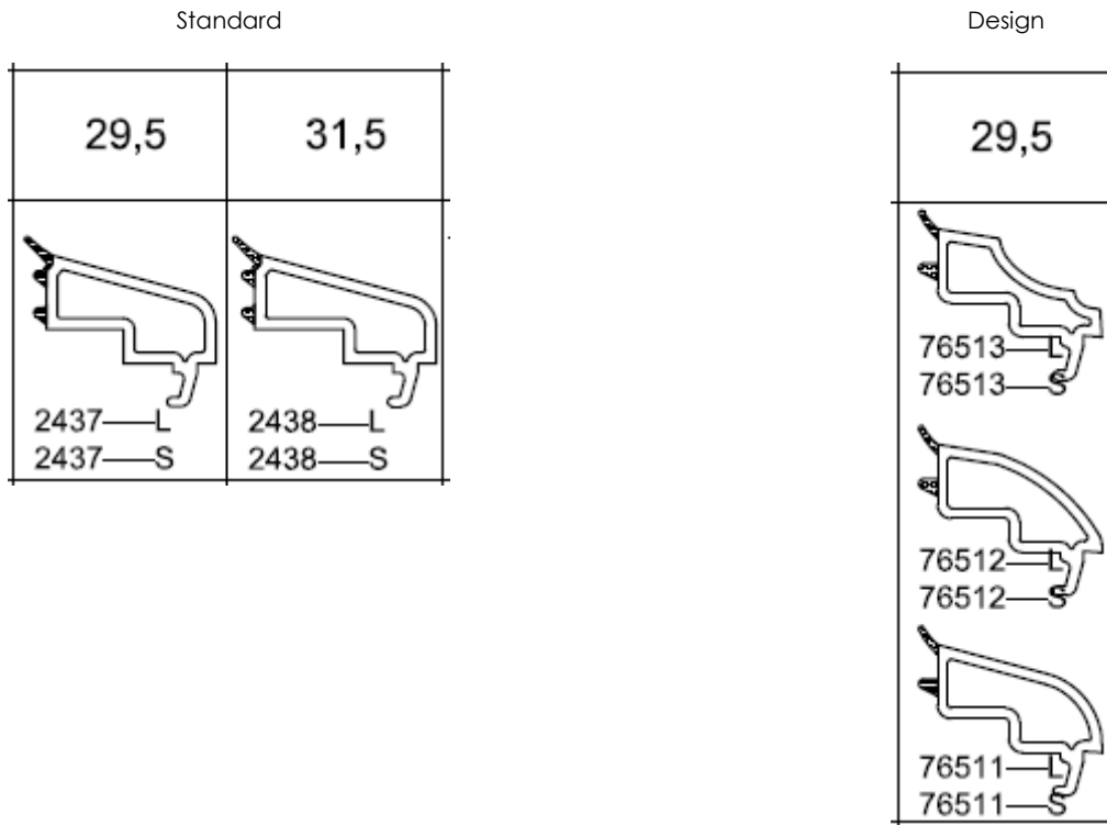
Figure 5a : Variantes d'exécution des parcloses
