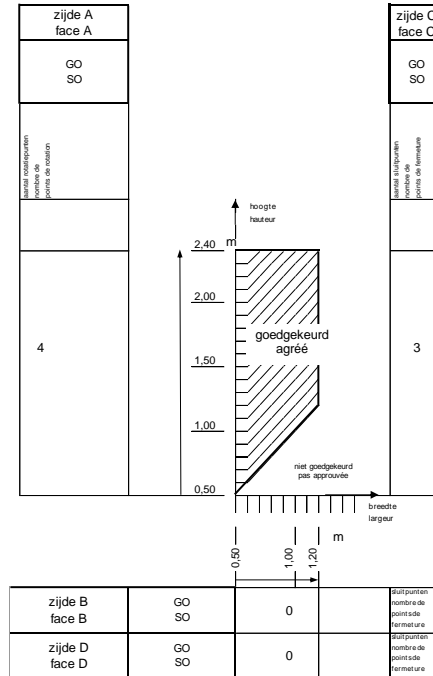
Beslagdiagram
