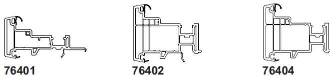
Figuur 3: Versterkingsprofielen
