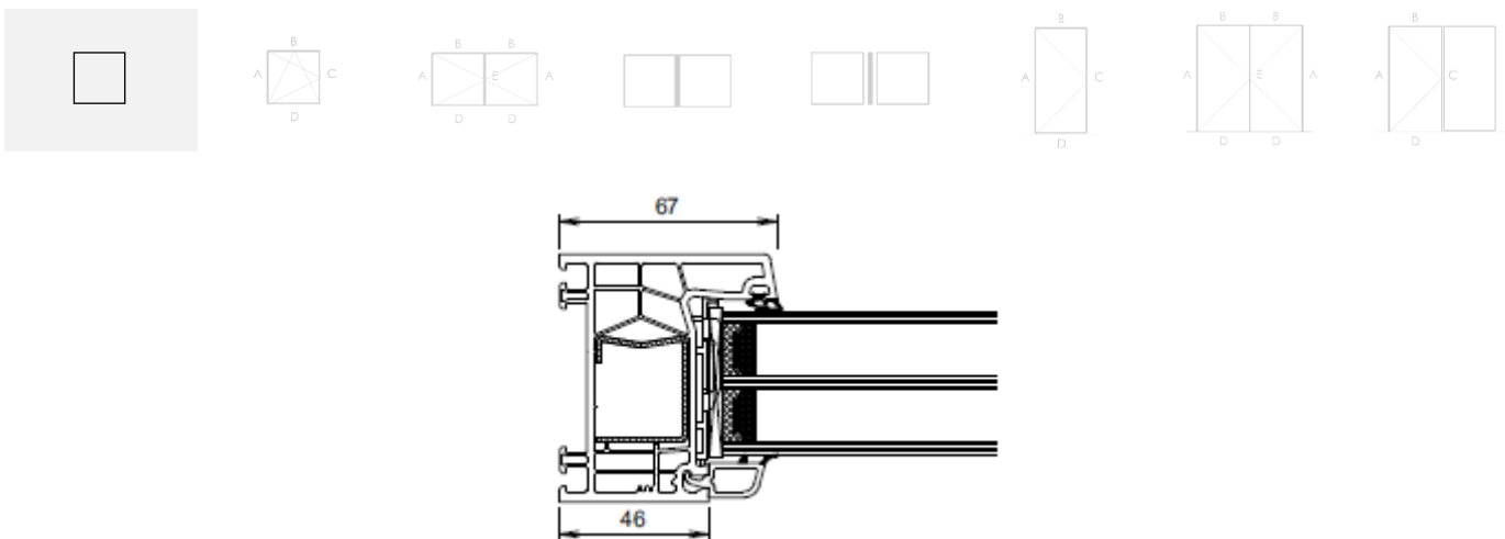
Figuur 7a: Typesnede vast venster
