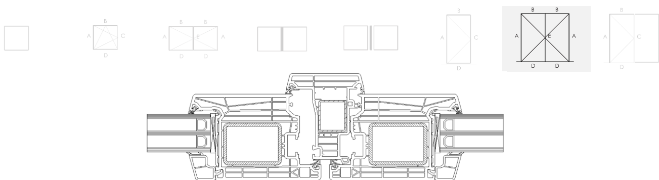
Figuur 8c: Typesnede samengestelde deur
