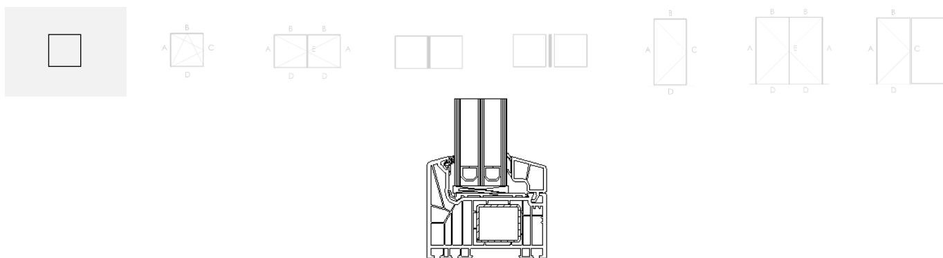
Figuur 7a: Typesnede vast venster
