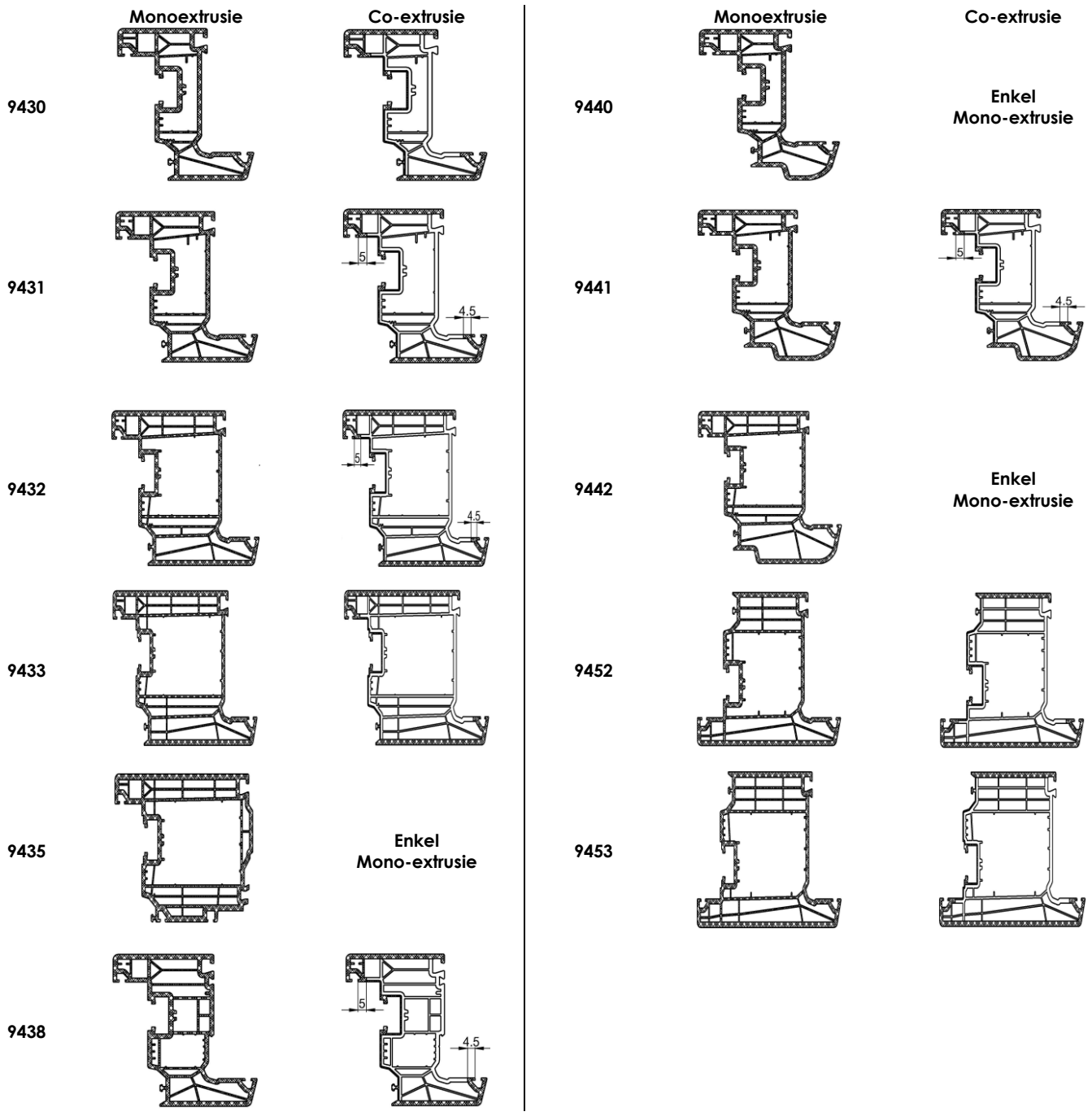
Figuur 2b: Vleugelprofielen
