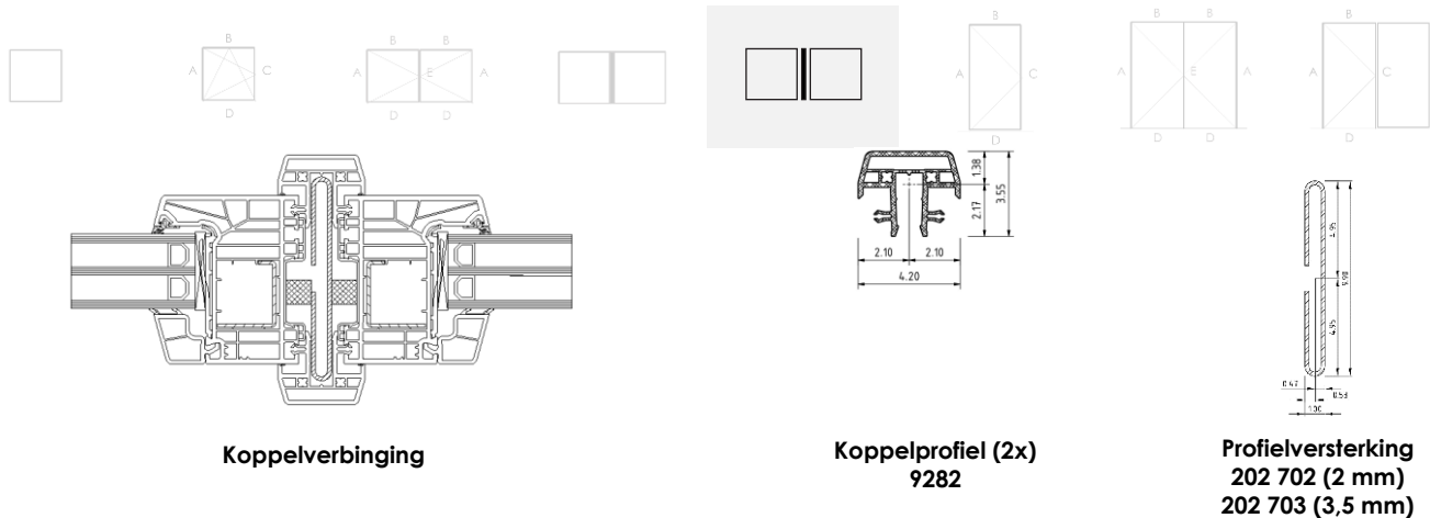
Figuur 8a: Typesnede enkele deur (met aanslagprofiel)
