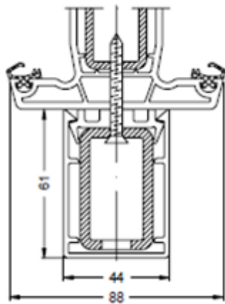
Figuur 5.c: Aanvullende profielen gecombineerd Aluminium/PVC - deurdorpels
