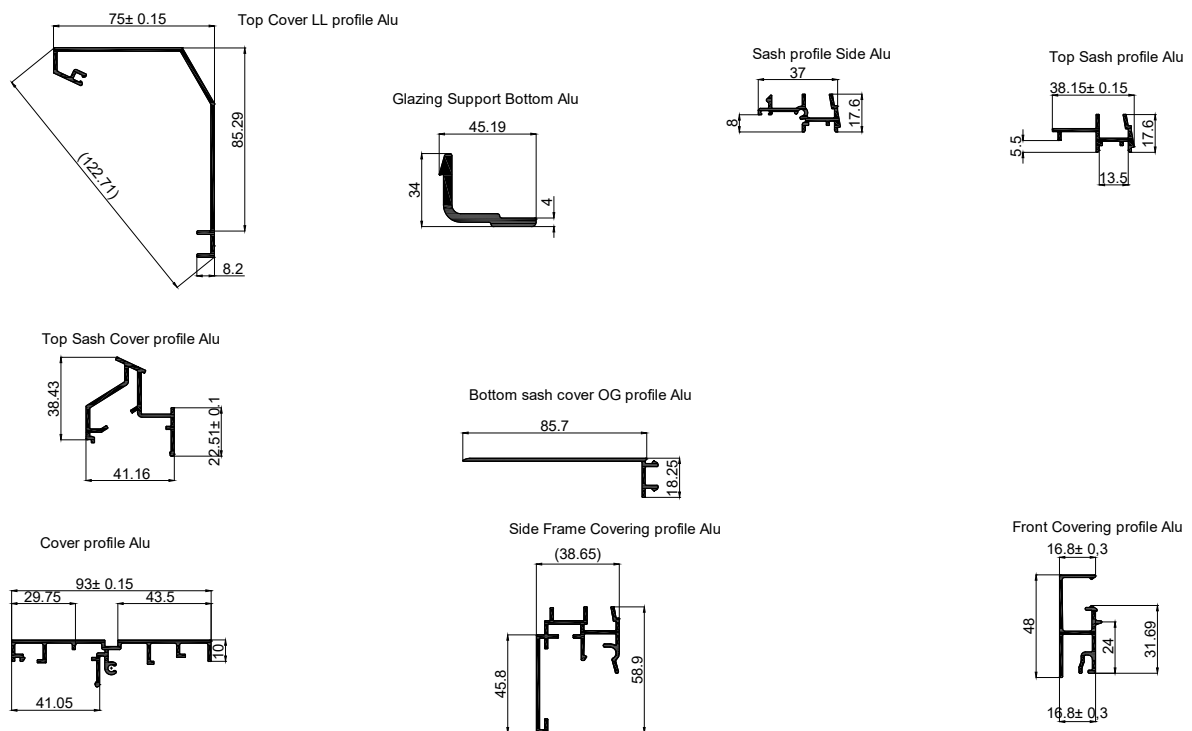
Figuur 4 – Aluminiumprofielen
