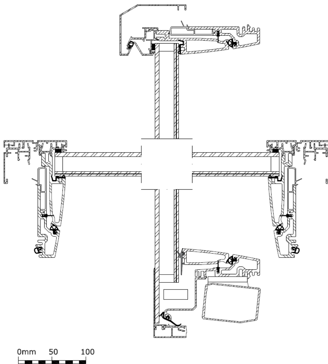
Figuur 1 – Doorsneden modulaire lichtstraat met opengaand kader
