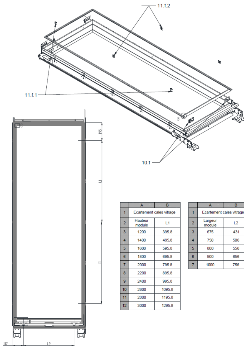
Figuur 6 – Positie van de glassteunblokken
