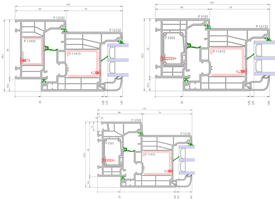
Figure 7c: Coupe-type de fenêtre à double ouvrant avec maillair
