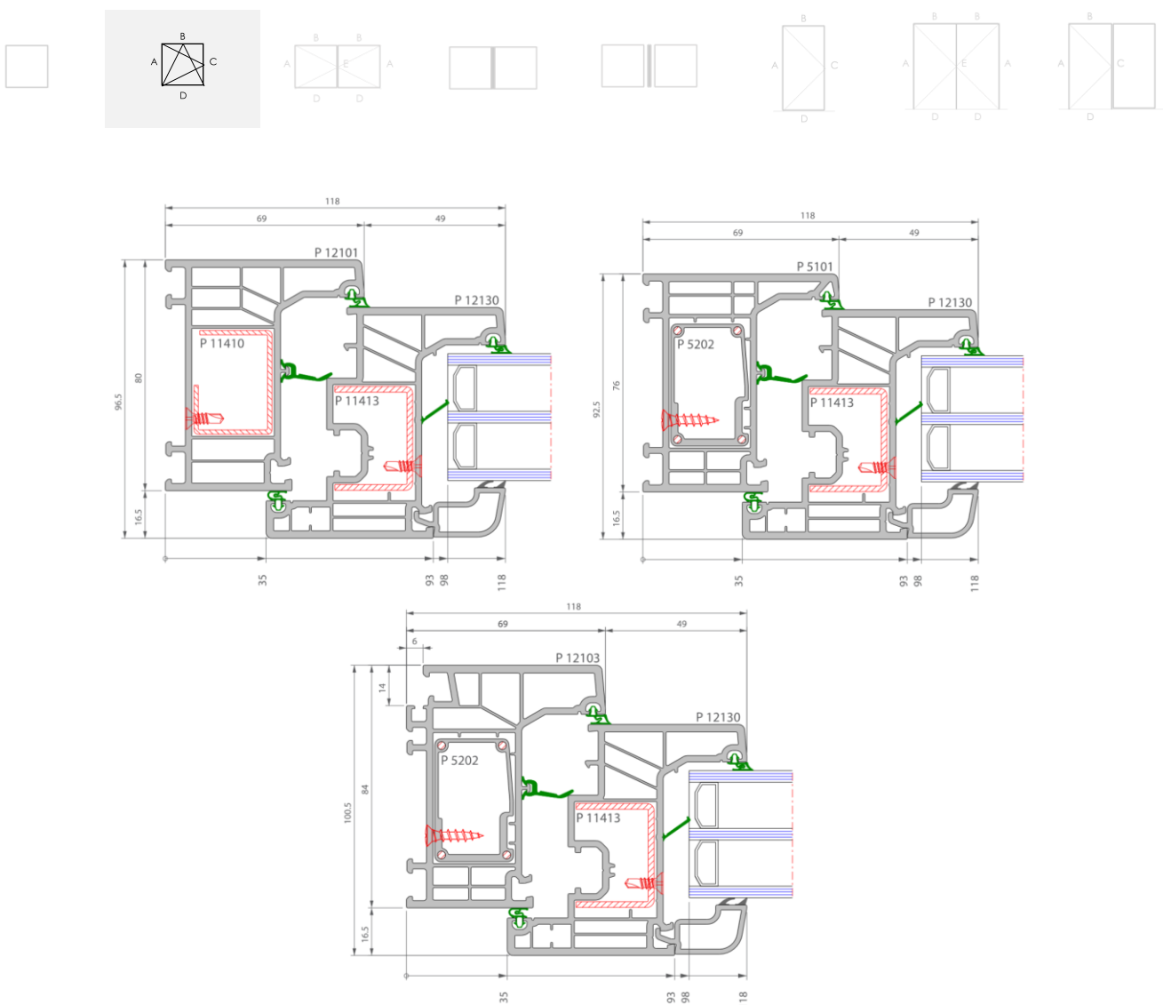
Figure 7b: Coupe-type de fenêtre oscillo-battante
