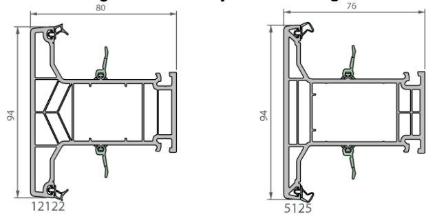
Figuur 2c: Tussenstijlen en dwarsregels
