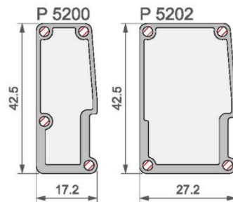
Figuur 3b – Thermische versterkingsprofielen
