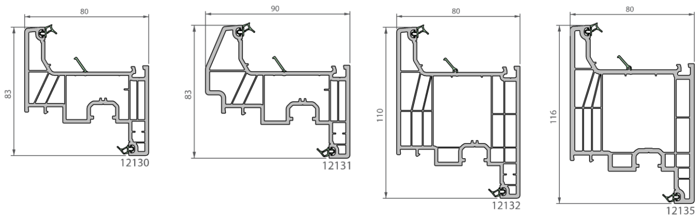
Figuur 2c: Tussenstijlen en dwarsregels
