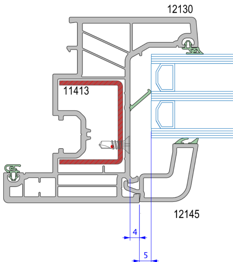
Figuur 9 - Convectiescheiding in de glasspanningsbodemplaat
