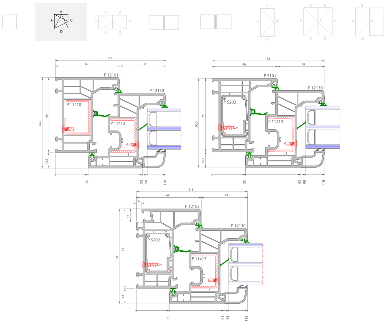
Figuur 7b: Typesnede draai-kip venster
