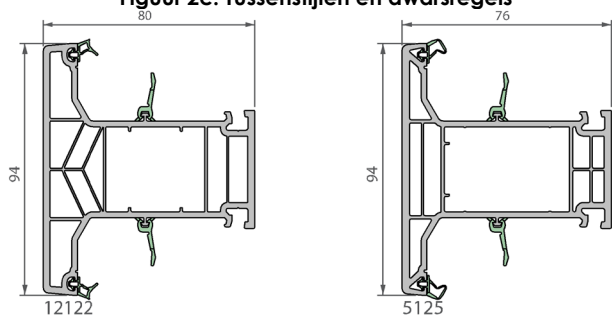
Figuur 2c: Tussenstijlen en dwarsregels
