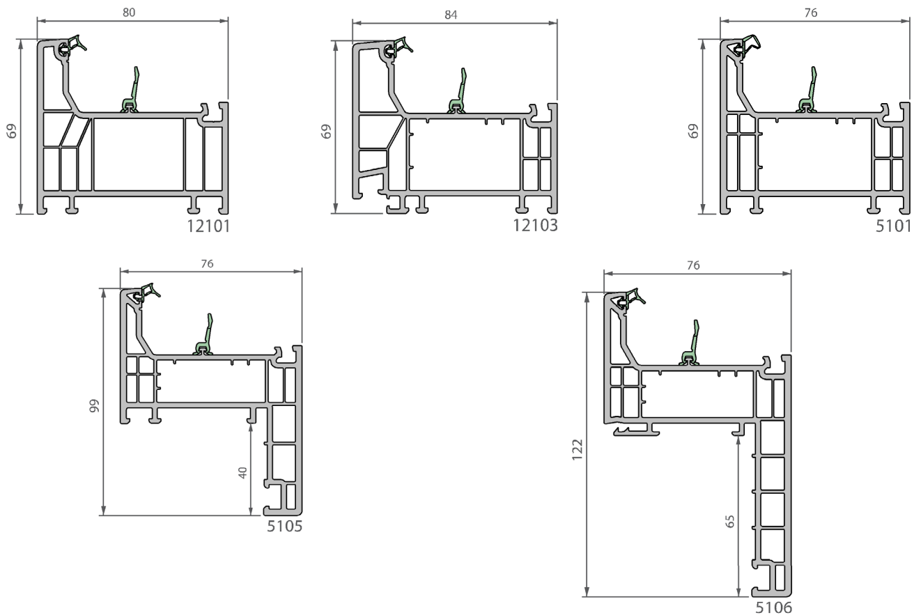
Figuur 2b: Vleugelprofielen
