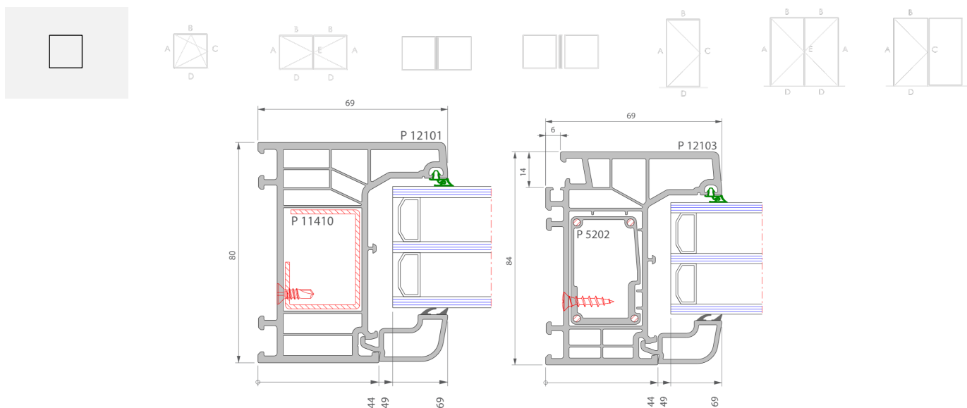
Figuur 7a: Typesnede vast venster
