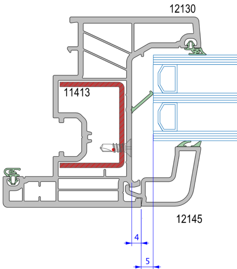
Figuur 9 - Convectiescheiding in de glassponningbodem
