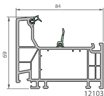
Figuur 2a: Kaderprofielen
