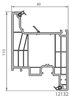
Figuur 2b: Vleugelprofielen
