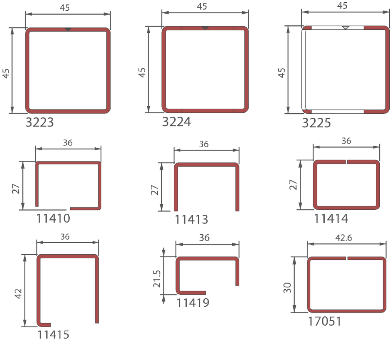
Figuur 3b – Thermische versterkingsprofielen
