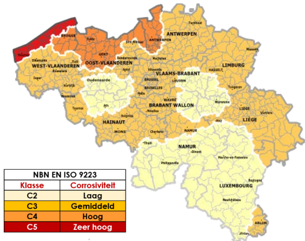
Fig. 1: Geografische agressiviteitszones
