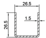
Figuur 3: Versterkingsprofielen
