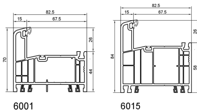
Figuur 2a: Kaderprofielen
