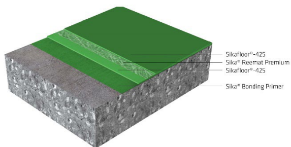
Fig. 1– SIKAFLOOR®-425 Waterdichtingssysteem
