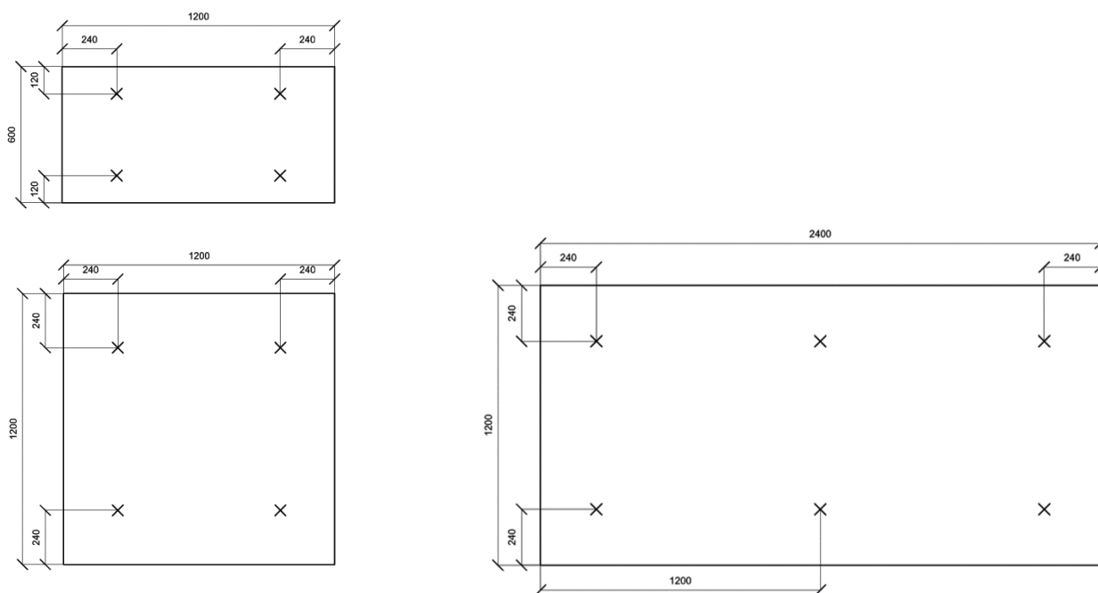
Fig. 1 – Plaatsingspatronen voor de mechanische bevestigingen
