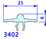
Figure 5.d : Profilés de seuil
