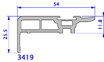
Figure 5.b: Profilés auxiliaires sans fonction de résistance
