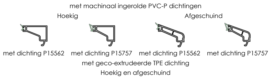
Figuur 5a: Uitvoeringsvarianten glaslatten
