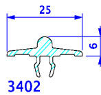
Figuur 5.d : Dorpelprofielen
