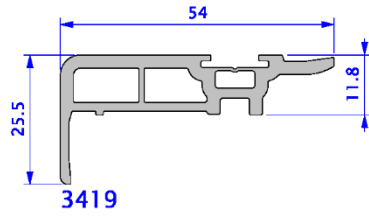
3419 Interlock en borstelhouder
