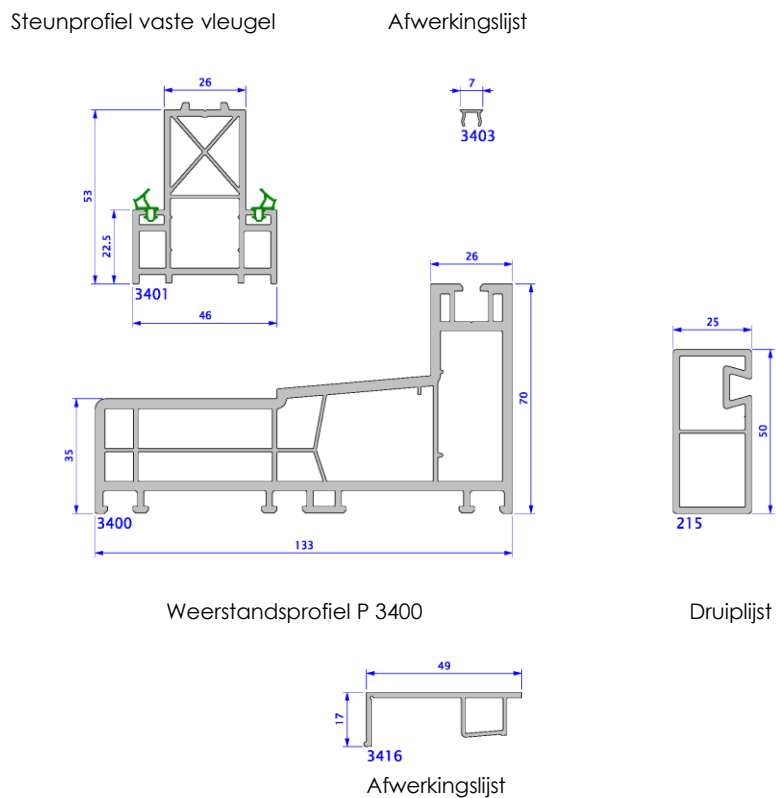
Figuur 2b: Vleugel en bijhorend PVC-U-profiel
