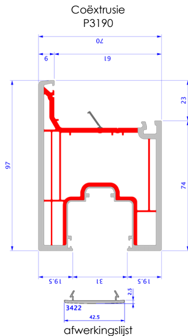
Figuur 2b: Vleugel en bijhorend PVC-U-profiel
