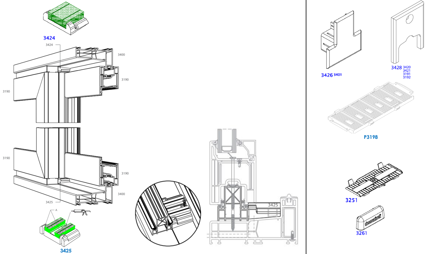
Figuur 6: Aanvullende kunststofstukken
