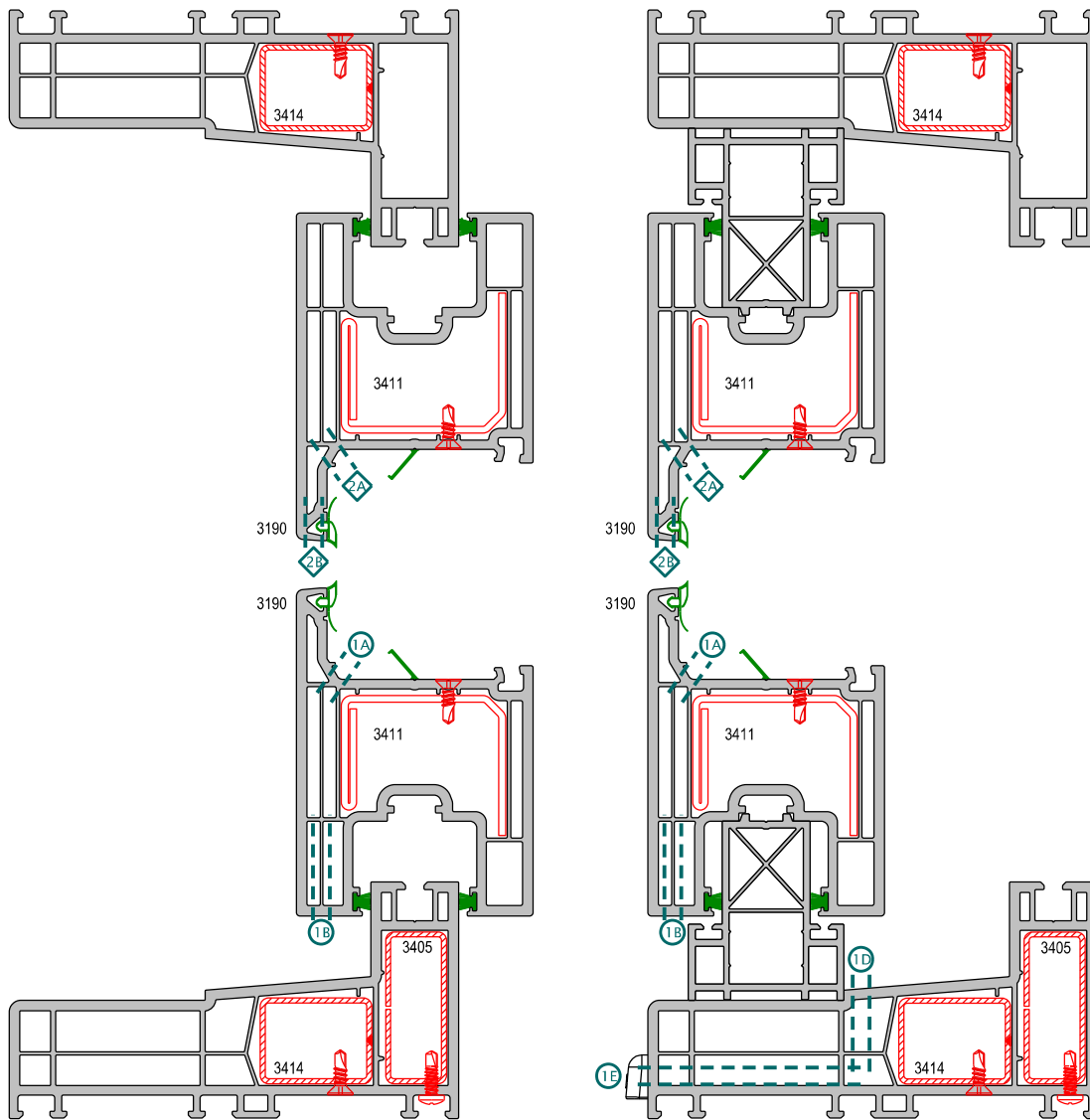
Figuur 8: Ontwatering en drukvereffening
