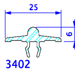
Figuur 5.c : Geleidingsrail
