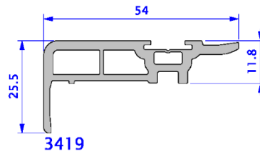
Figuur 5.b: Aanvullende profielen zonder weerstandsfunctie
