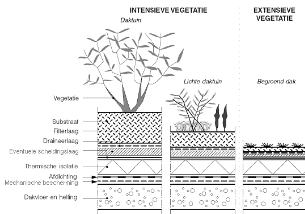
Fig. 2 – Omkeerdak opbouw
