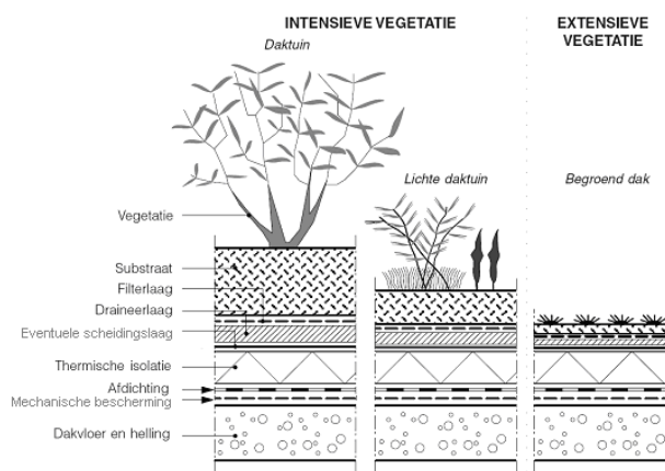
Fig. 2 – Omkeerdak opbouw
