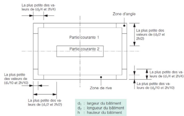
Fig. 3 – Détermination des zones d'angle (a), de rive (r) et des parties courantes (t)
