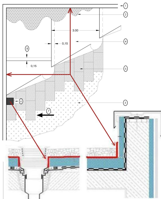
Fig. 2 – Mise en œuvre du système RAVATHERM XPS MinK
