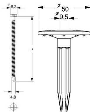
Fig. 2 – Schroef ZAHN ZDBK 4,8+ bevestigingstule ZAHN ZKSH ROUND
