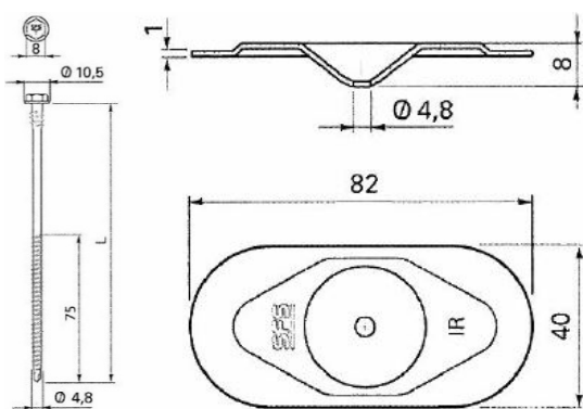
Fig. 1 – Schroef SFS IR2 + bevestigingsplaatje IR
