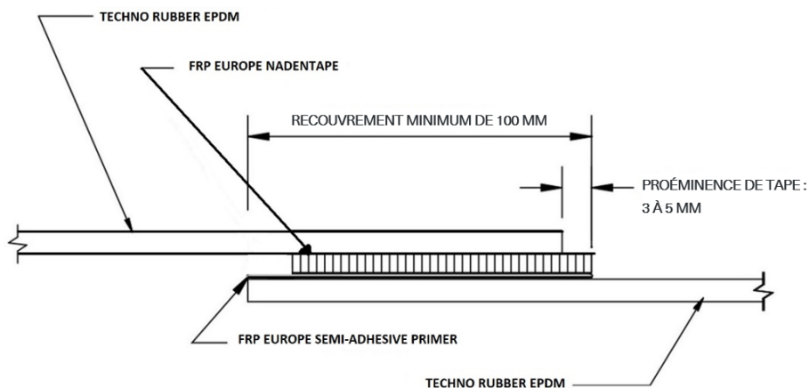
Fig. 1 – Raccords par recouvrement dans le sens longitudinal
