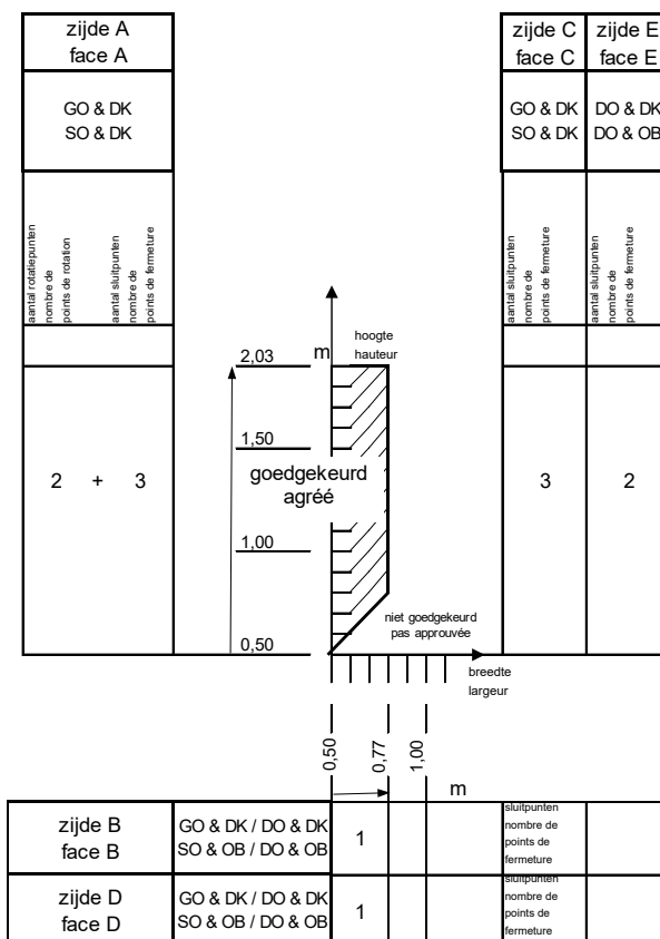
Beslagdiagram
