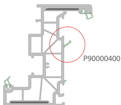
Figuur 10: Convectiescheiding P90000400
