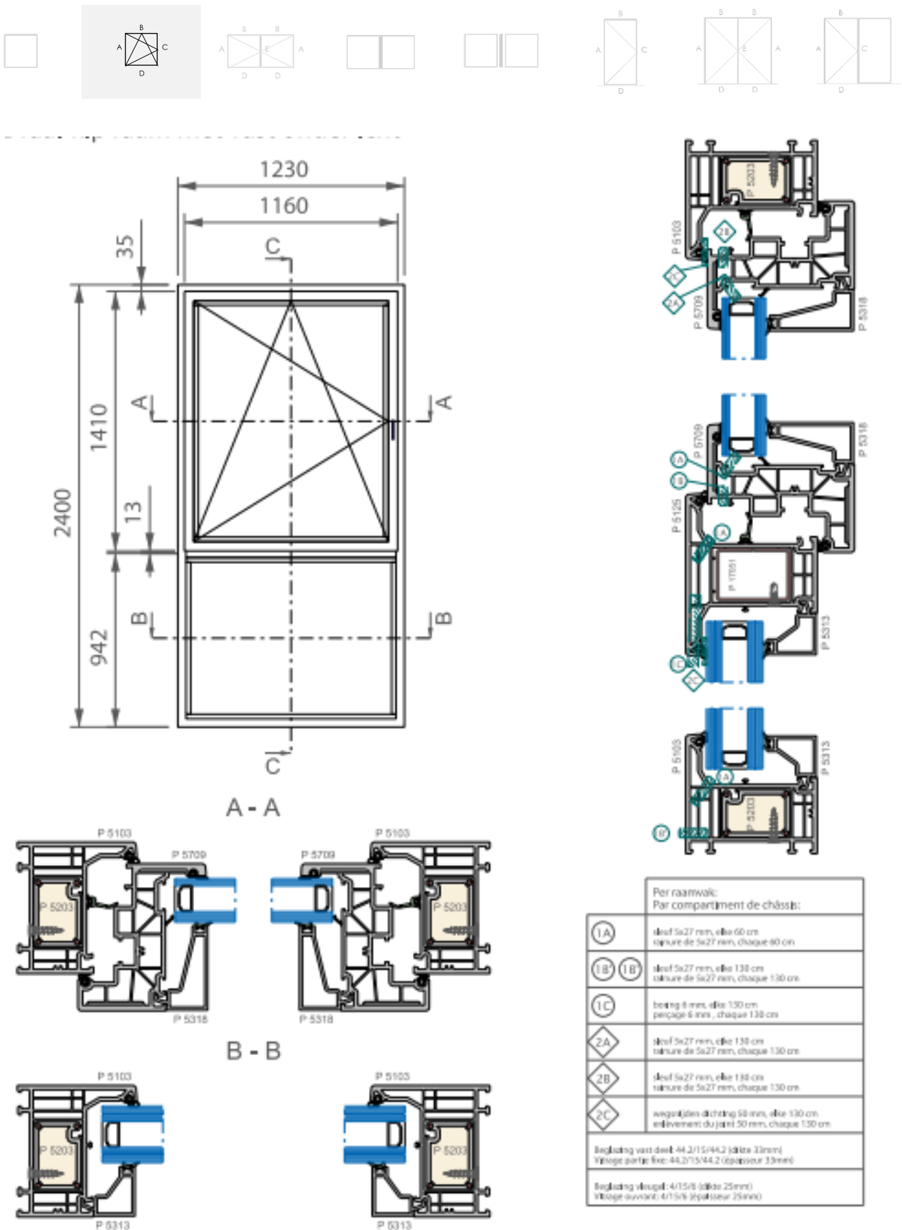
Figuur 7b: Typesnede draai-kip venster
