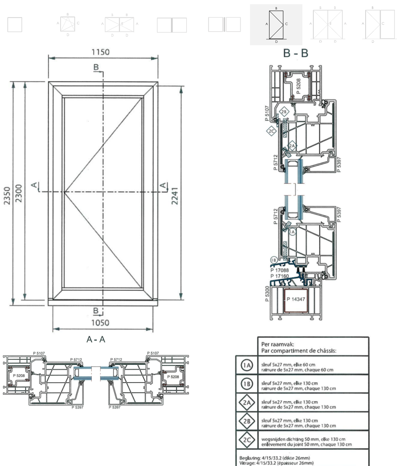
Figuur 8.a: Typesnede enkele deur
