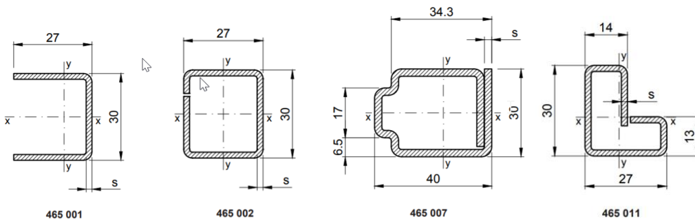
Figuur 3a – Versterkingsprofielen uit gegalvaniseerd staal
