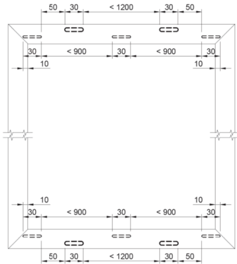
Afwatering en verluchting vleugel
