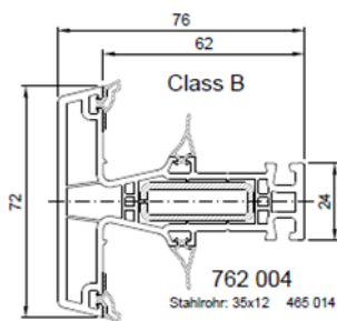
Figuur 2d: Mechanische T-verbinding
