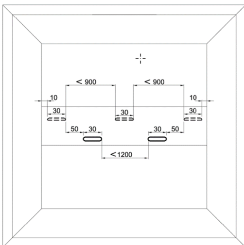
Afwatering en verluchting T-profiel
