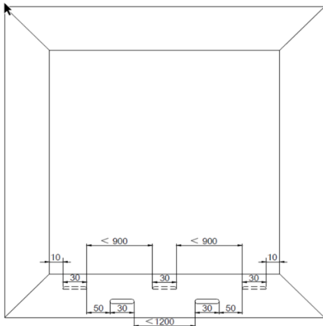
Afwatering en verluchting vleugel
