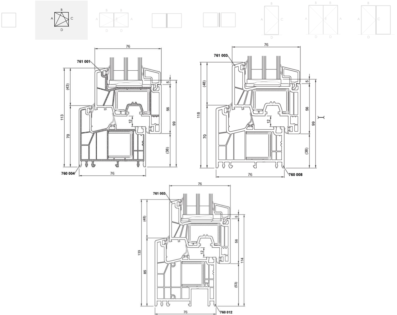
Figuur 7b: Typesnede draai-kip venster
