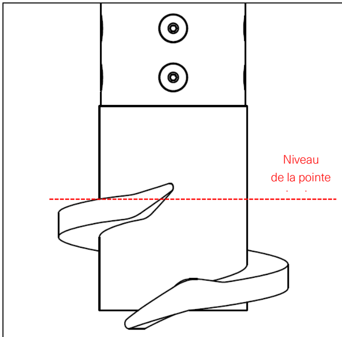
Fig. 1 : Dessin technique de la tarière (type Olivier)
