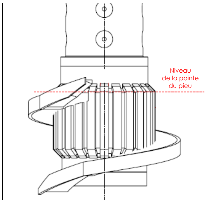
Fig. 1 : Dessin technique de la tarière prise en considération (type Helix)
