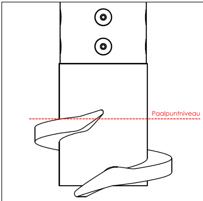
Fig. 1 : Technische schets van de boorkop (type Olivier)
