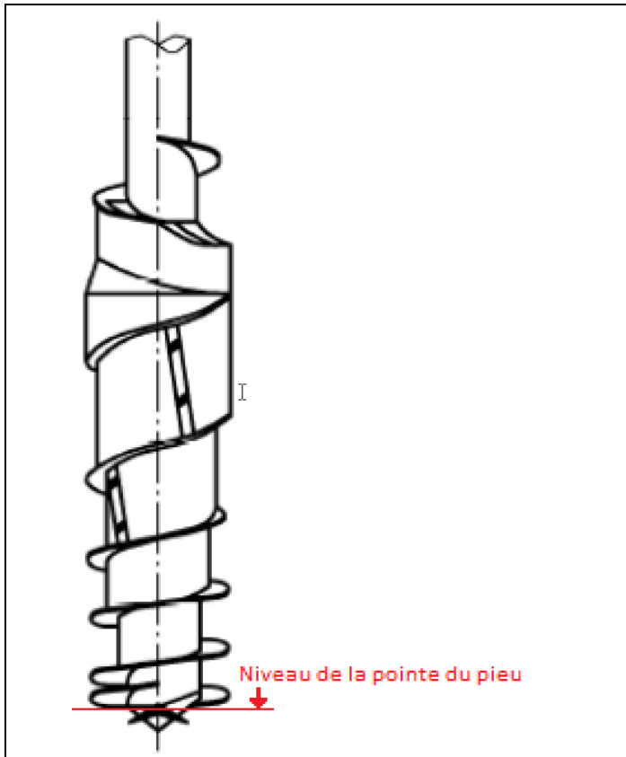
Fig. 1 : Dessin technique de la tarière à refoulement (type Omega)
